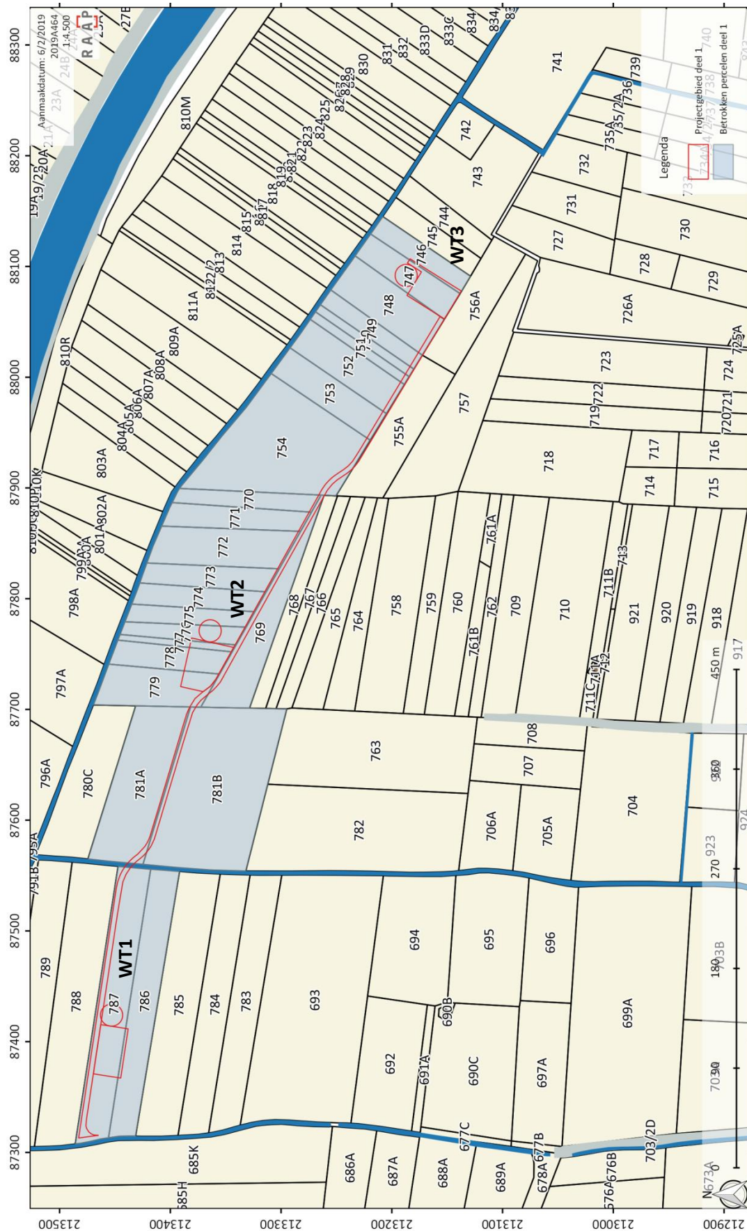
figuur 2 Kadasterplan met projectie van de betrokken percelen van deel 1 en aanduiding van de voorziene uitgravingen en de individuele nummers van de windturbines (bron: Grootchalig Referentiebestand Vlaanderen, AGIV)
