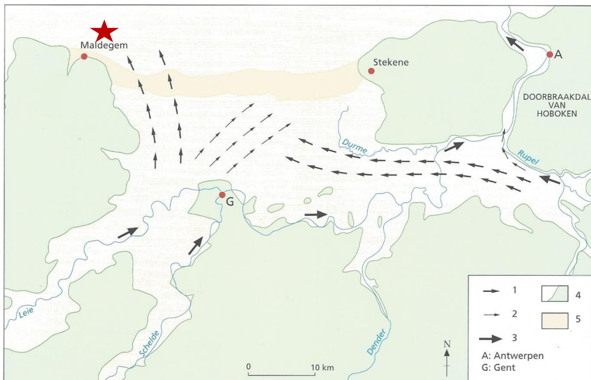
figuur 8 De morfologie van de Vlaamse Vallei met aanduiding van het verloop van de rivieren in verschillende periodes en de dekzandrug Maldegem-Stekene. (Van Strydonck & De Mulder, 2000, 21, fig. 8). De situering van het plangebied is met een ster weergegeven.
