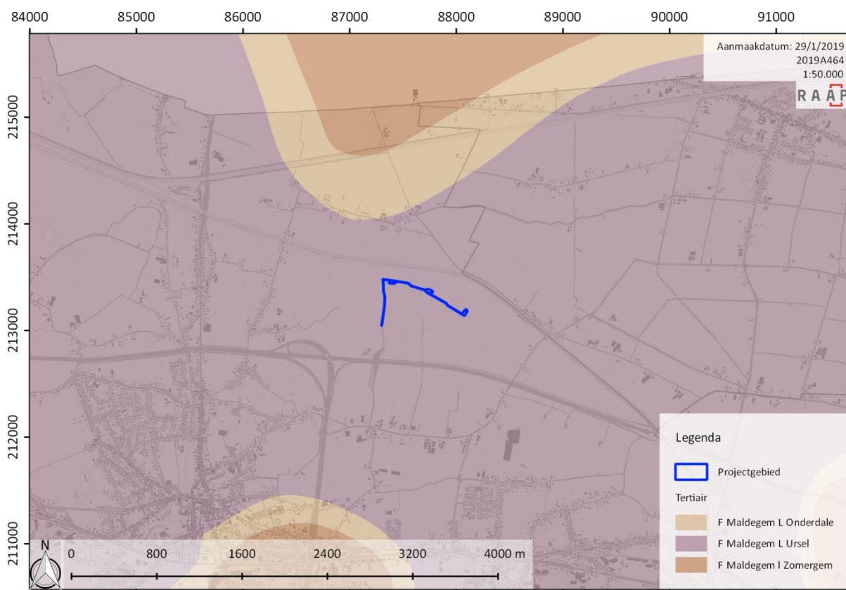
figuur 10 Tertiair geologische kaart met projectie van het plangebied (bron: DOV, Grootchalig Referentiebestand Vlaanderen, AGIV)
