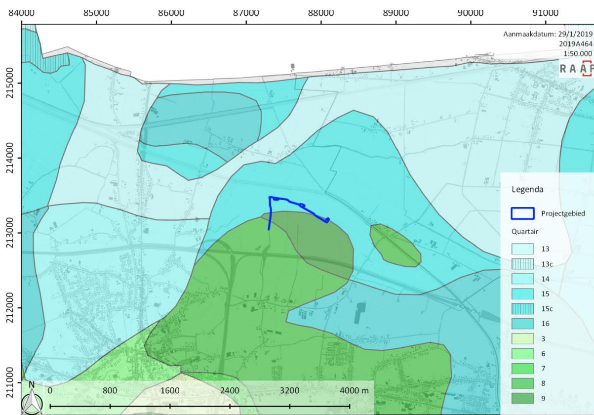
figuur 11 Quartair geologische kaart met projectie van het plangebied (bron: DOV, Grootchalig Referentiebestand Vlaanderen, AGIV)
