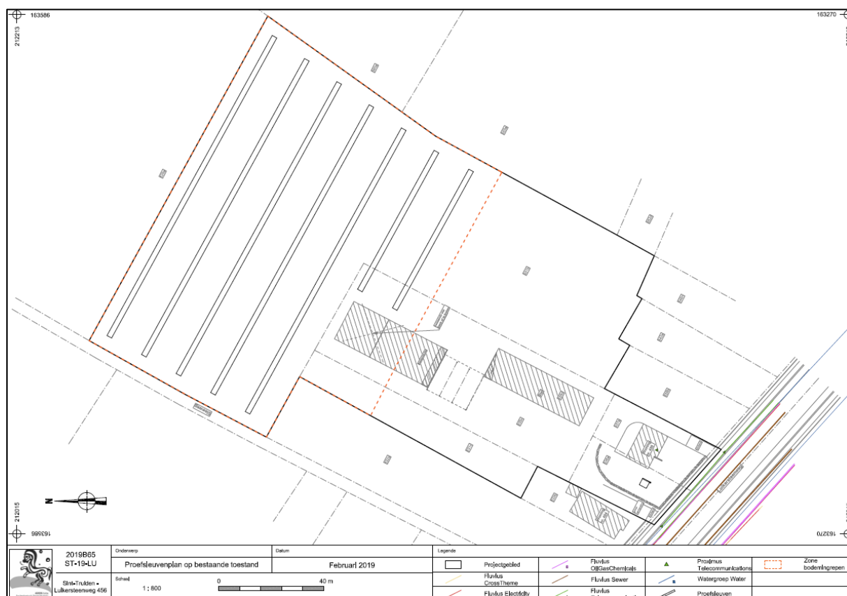
Afb. 33: Sleuvenplan op bestaande toestand met aanduiding van het onderzoeksgebied (zwart) en de geplande sleuven in het zwart (Bron: Aron bvba, digitaal plan, dd. 13/02/2019, aanmaatschaal 1:800, 2019B95).
