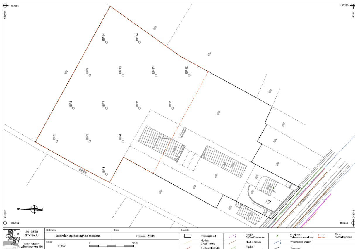
Afb. 31: Boorplan met aanduiding van de boorpunten en het projectgebied (zwart), de zone voor vervolgonderzoek (oranje) op bestaande toestand (BT) ((Bron: Aron bvba, digitaal plan, dd. 13/02/2019, aanmaatschaal 1.800, 2019B65).
