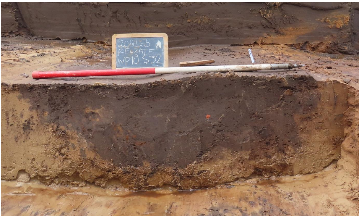
Figuur 27 Coupe op gracht S32.
