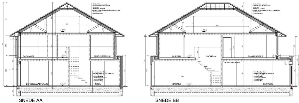
Figuur 3.5 : Doorsnede gepland bouwproject.
