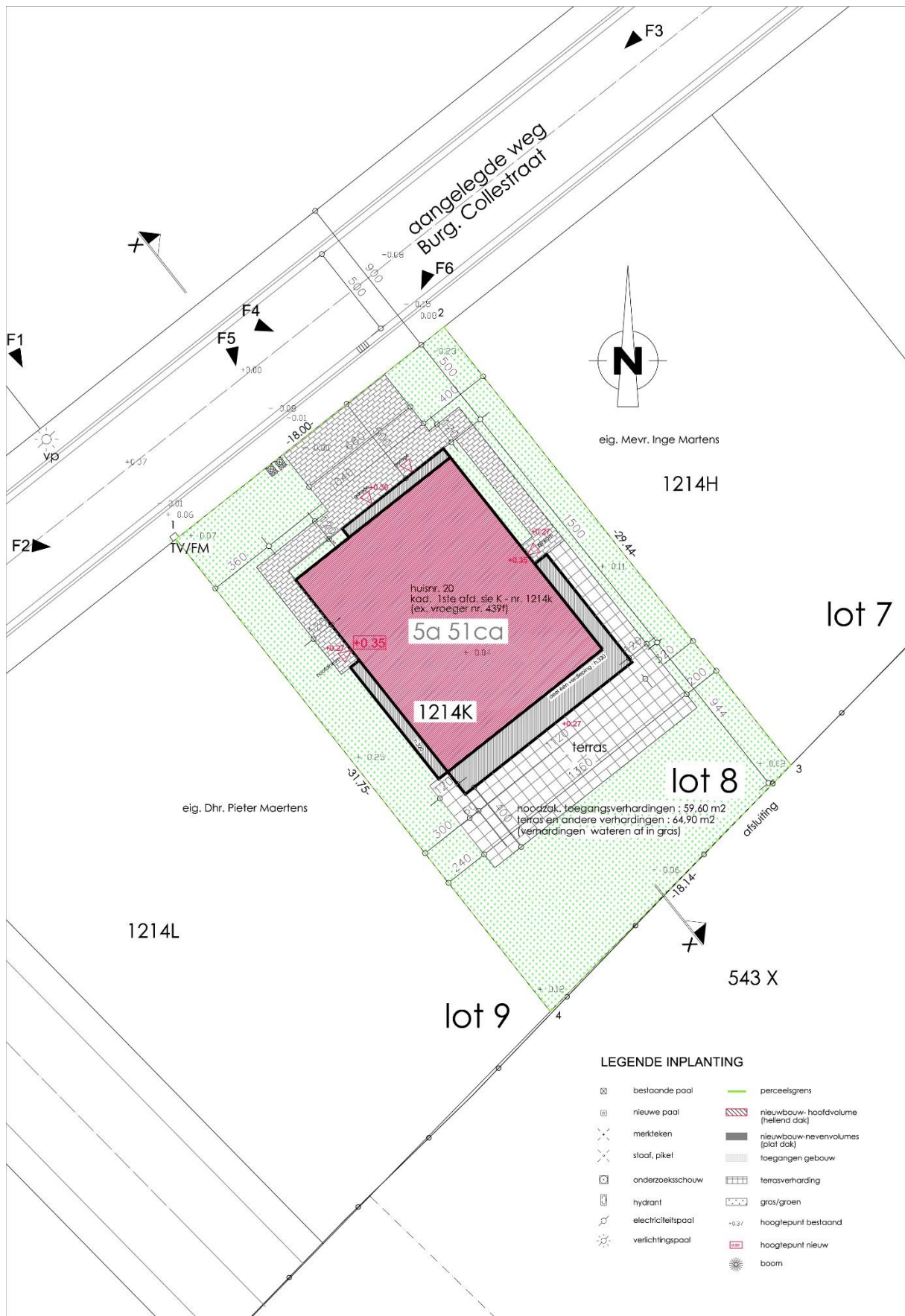
Figuur 3.2 : Grondplan van het geplande bouwproject.
