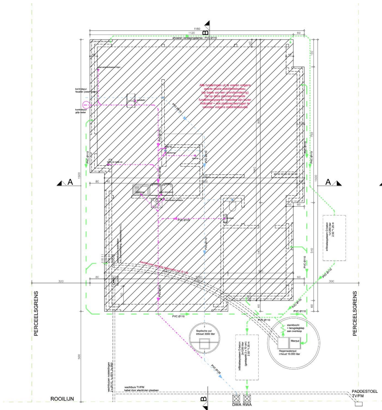
Figuur 3.3 : Funderings- en rioleringsplan van het geplande bouwproject.
