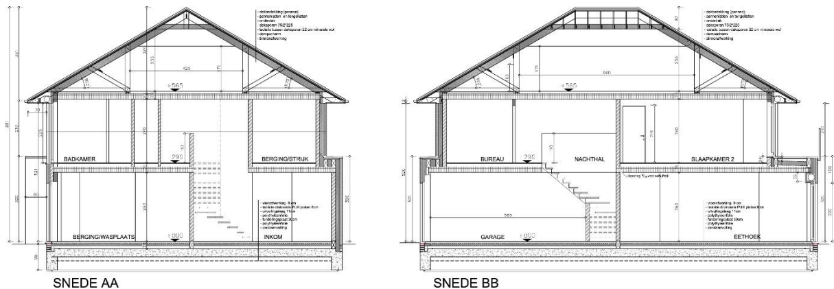
Figuur 7d : Doorsnede gepland bouwproject.
