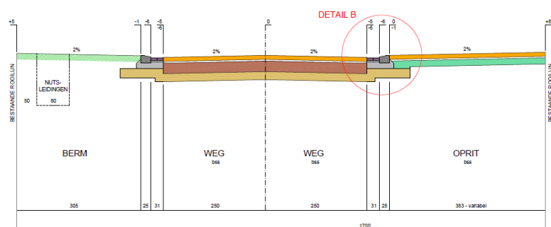
TYPEDWARSPROFIEL C-C
