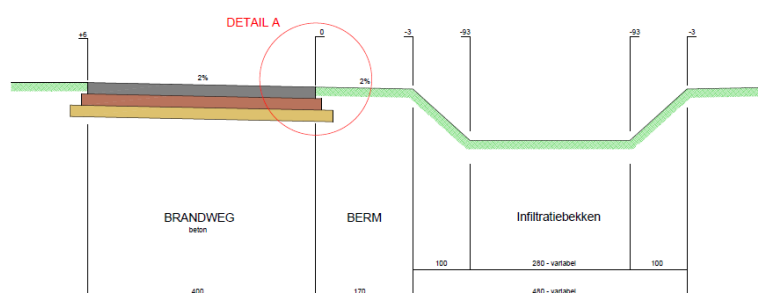
TYPEDWARSPROFIEL D-D
