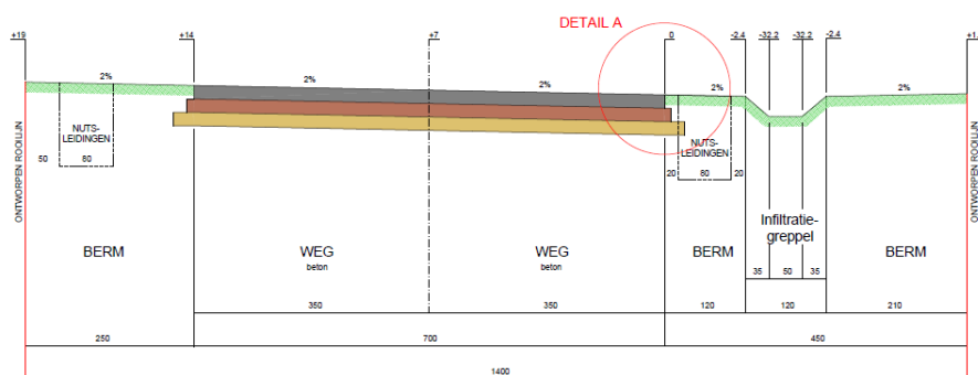
TYPEDWARSPROFIEL A-A
