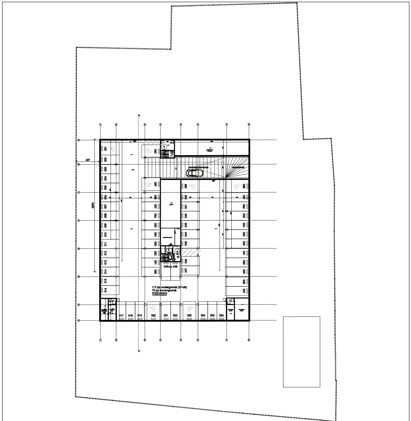
Figuur 32: Plan van de ondergrondse infrastructuur niveau -2 (© Bontinck Architecture & Engineering NV)
