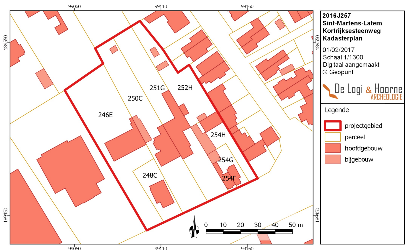
Figuur 30: Kadasterkaart met aanduiding van het projectgebied en perceelsnummers (© Geopunt)
