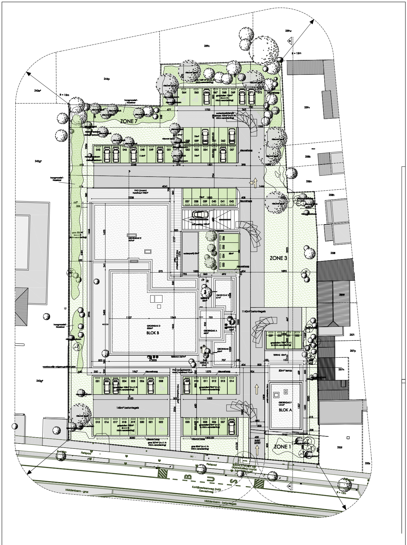
Figuur 31: Plan van de bestaande toestand en de geplande werken (© Bontinck Architecture & Engineering NV)
