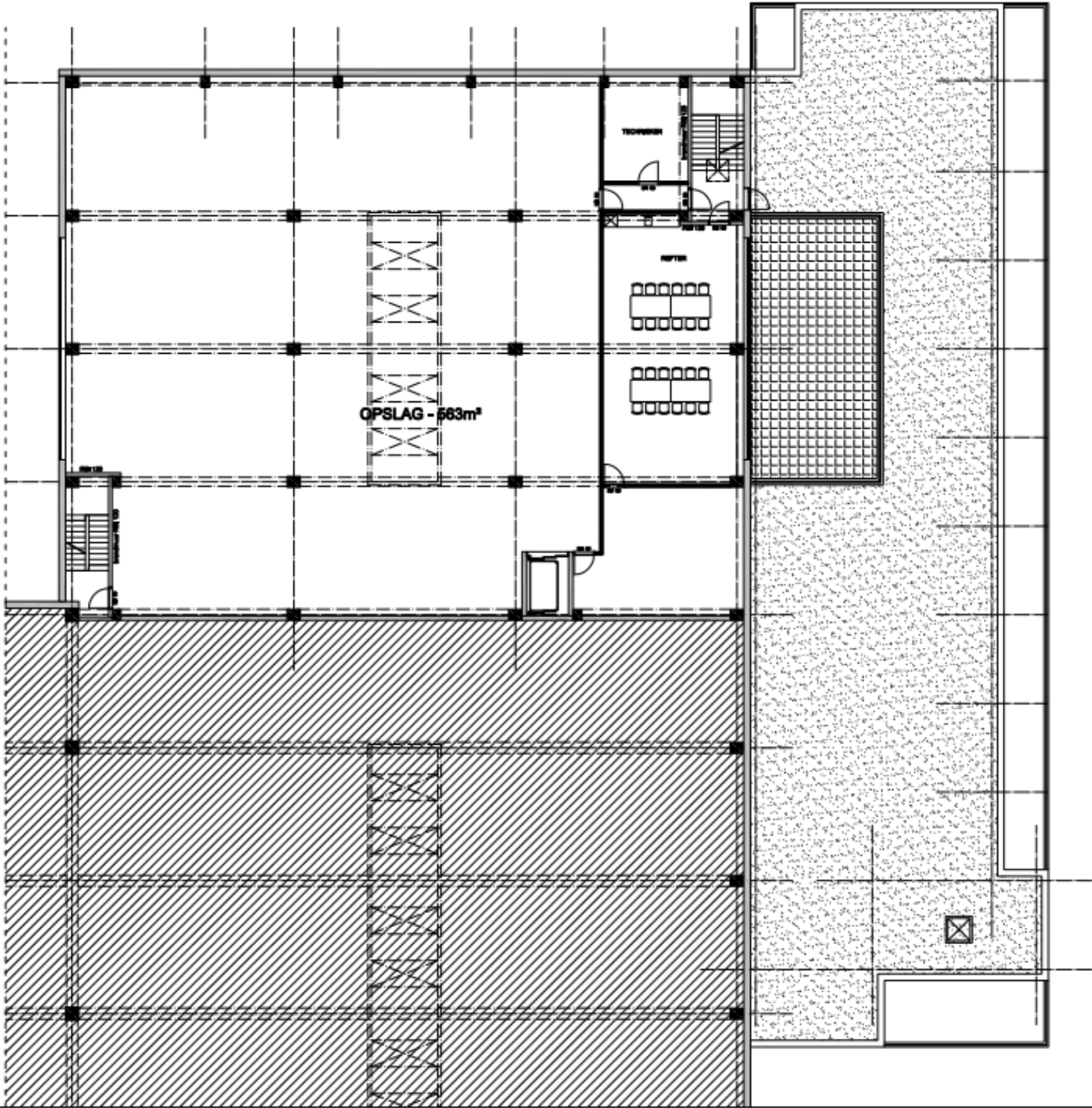
GRONDPLAN - niv +2
