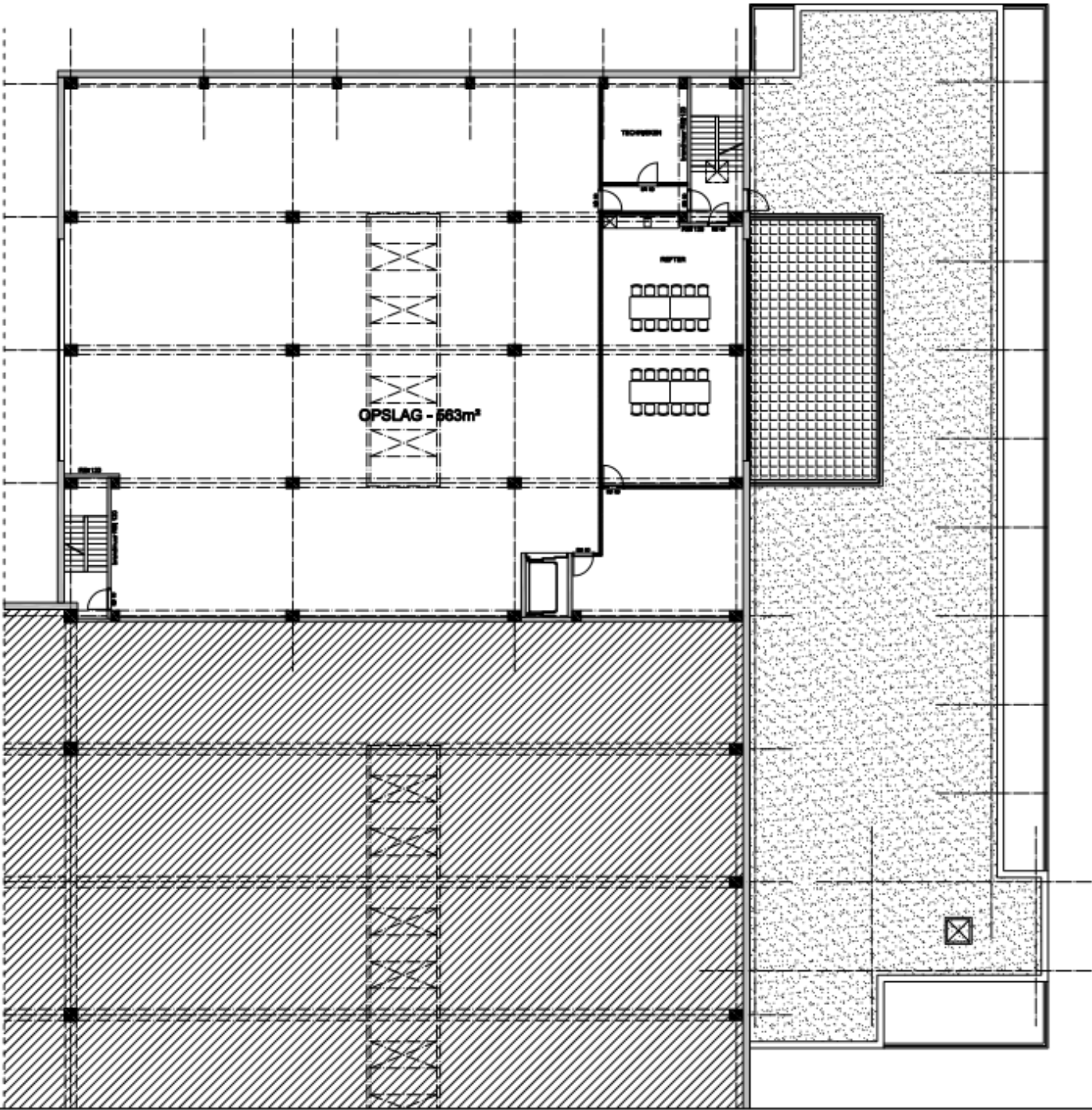
GRONDPLAN - niv +2
