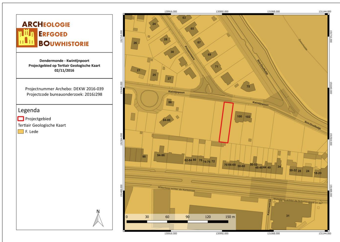
Figuur 22: Situering van het onderzoeksgebied op de Tertiairgeologische kaart (DOV, 2016).
