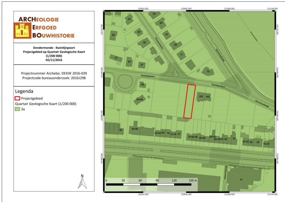
Figuur 23: Situering van het onderzoeksgebied op de Quartairgeologische kaart 1/200.000 (DOV, 2016).
