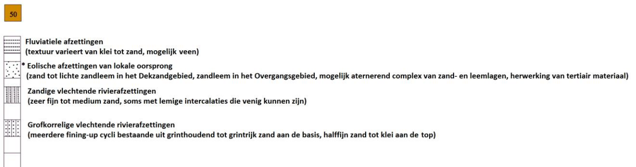
Figuur 26: Uitleg van het type volgens de Quartairgeologische kaart, schaal 1:50.000 (DOV, 2016).
