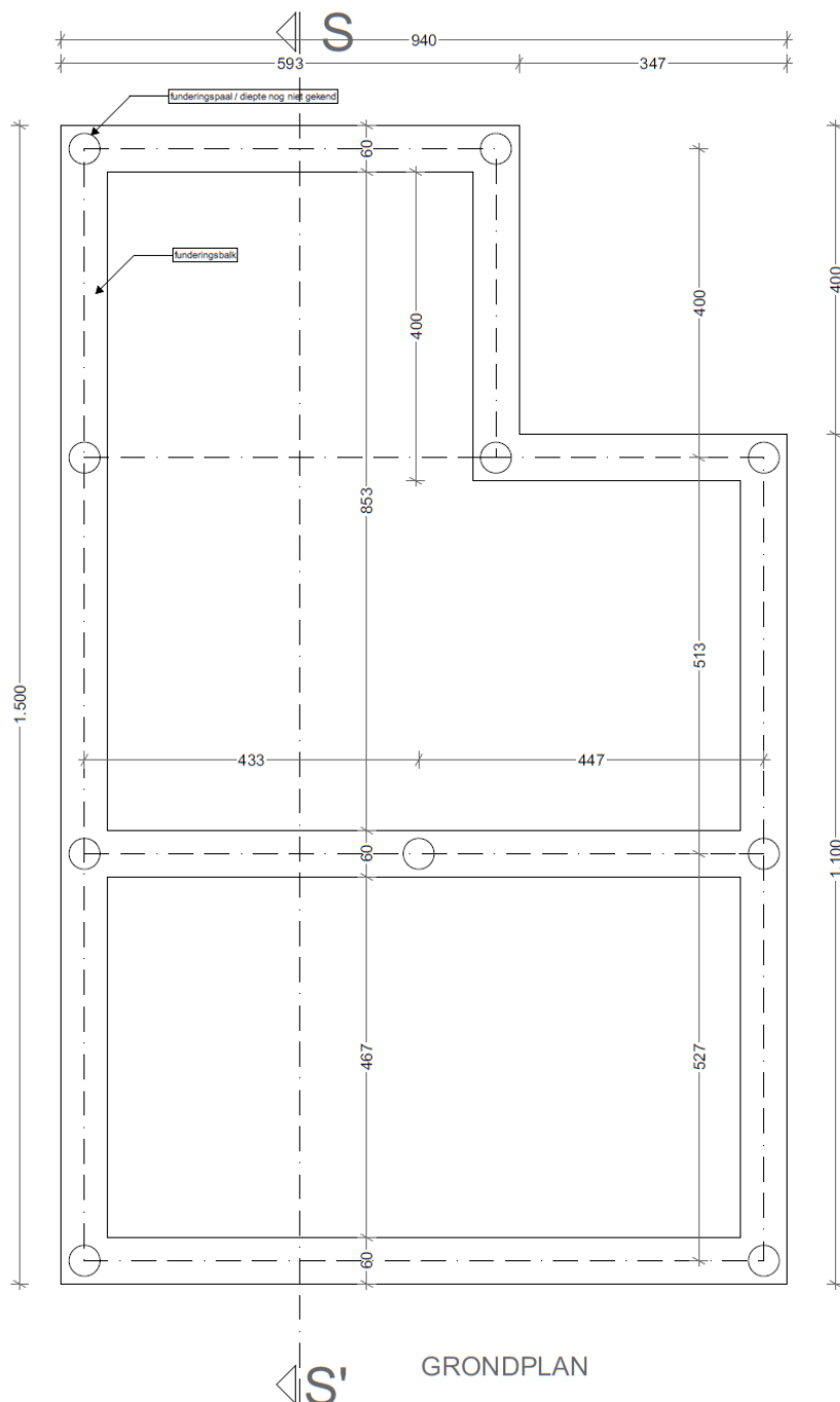
Figuur 15: Omvang van de geplande bodemingreep met aanduiding van de plaatsing van de funderingspalen- en balken (W.A.R.R.P. Architectenbureau bv-bvba, 2016).
