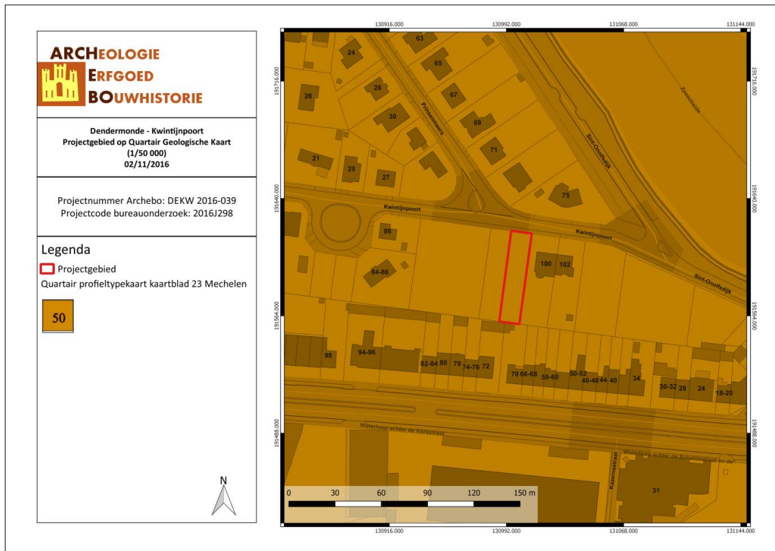
Figuur 25: Situering van het onderzoeksgebied op de Quartairgeologische kaart 1/50.000 (DOV, 2016).
