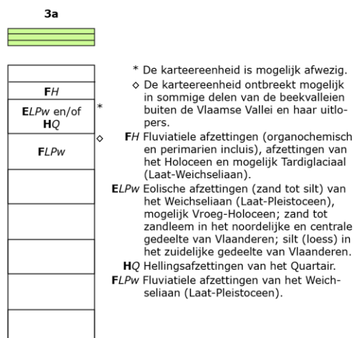
Figuur 24: Uitleg van het type volgens de Quartairgeologische kaart, schaal 1:200.000 (DOV, 2016).
