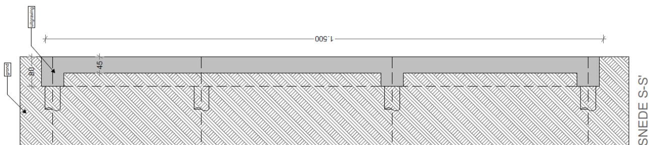
Figuur 16: Snede van de geplande bodemingreep (W.A.R.R.P. Architectenbureau bv-bvba, 2016).
