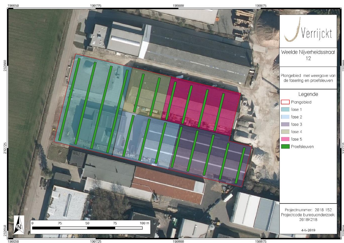
Figuur 4: Sleuvenplan
