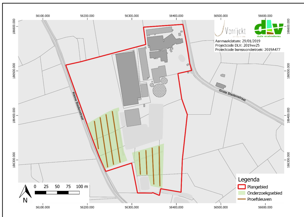
Figuur 3: Sleuvenplan
