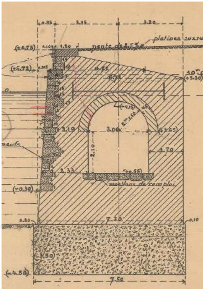
Figuur 6: Bestaande toestand kaaimuur Havenstraat (Bron: AGENTSCHAP MARITIEME DIENSTVERLENING en KUST).
