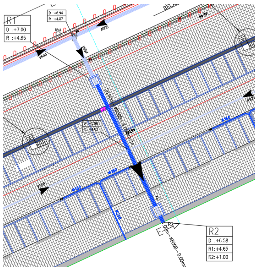
Figuur 10: Aanduiding nieuwe riolering (Bron: AGENTSCHAP MARITIEME DIENSTVERLENING en KUST).
