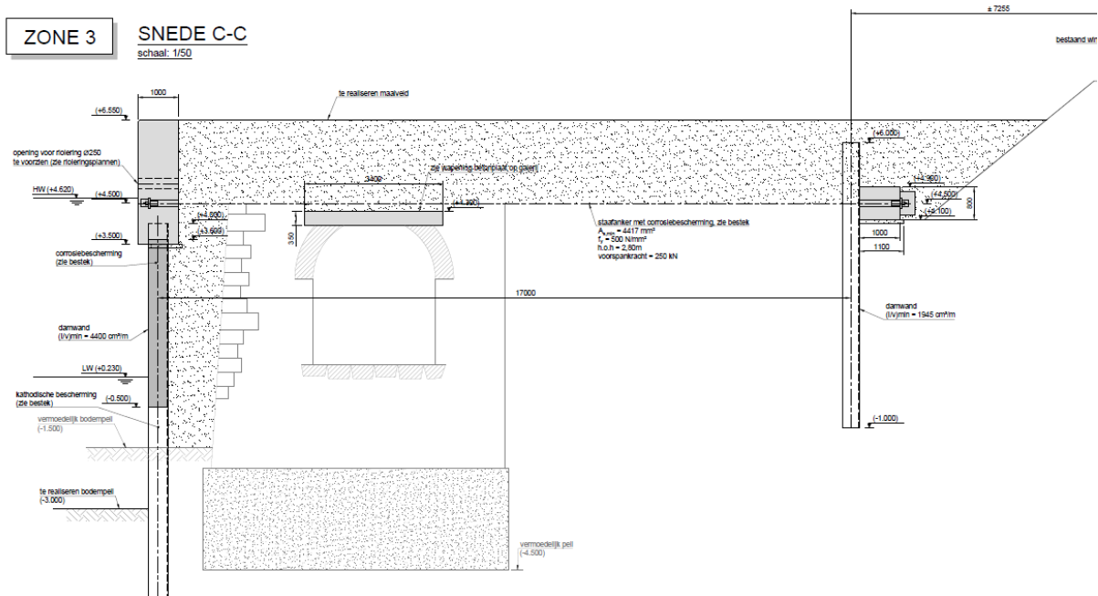
Figuur 11: Dwarsdoorsnede te realiseren kaaimuur Havenstraat (Bron: AGENTSCHAP MARITIEME DIENSTVERLENING en KUST).
