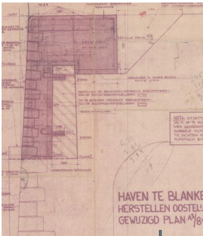
Figuur 7: Vernieuwing bovenbouw kaaimuur Franchommelaan (Bron: AGENTSCHAP MARITIEME DIENSTVERLENING en KUST).
