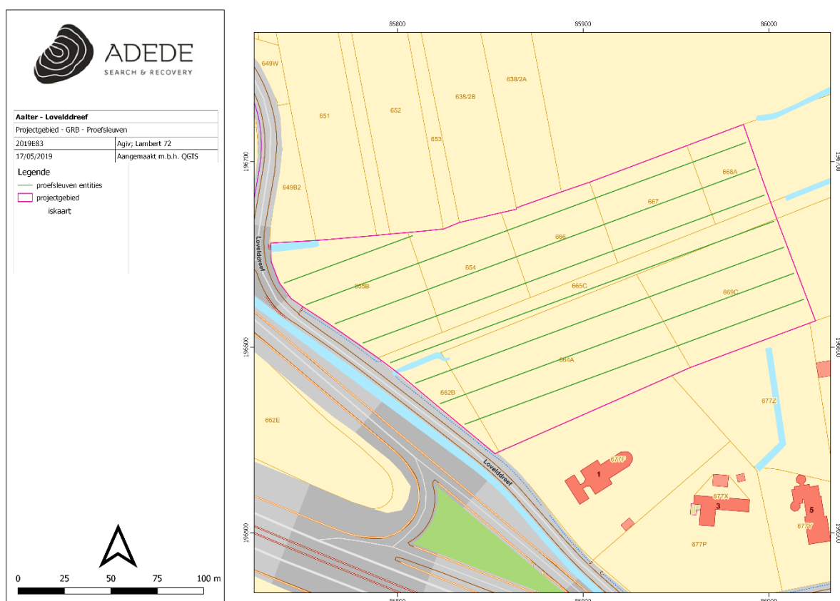
Figuur 3. Sleuvenplan
