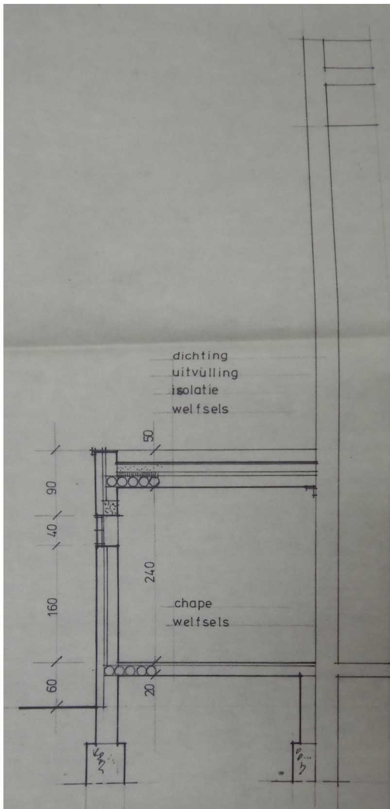
Fig. 4. Doorsnede van de aanbouw.
