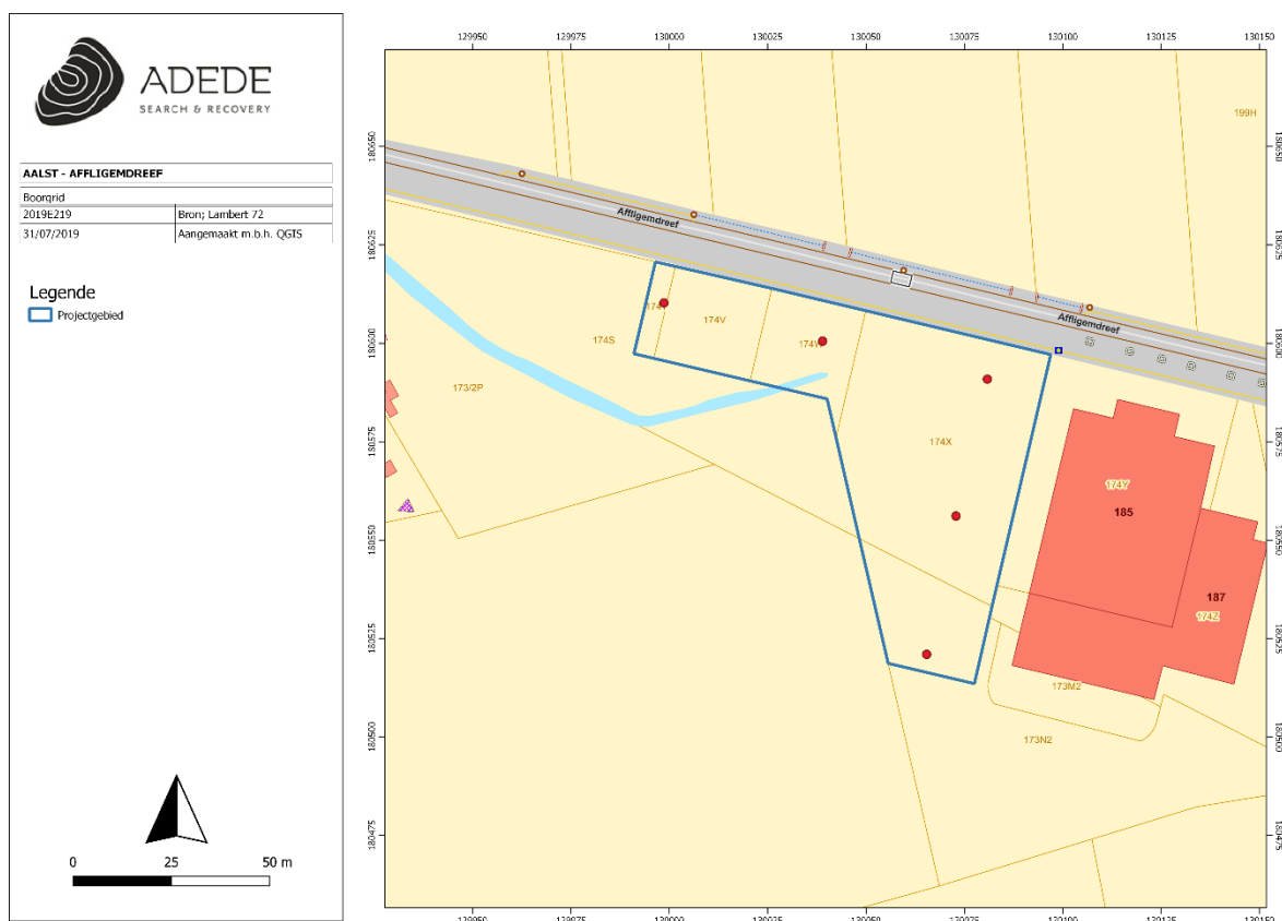
Figuur 2. Boorplan.
