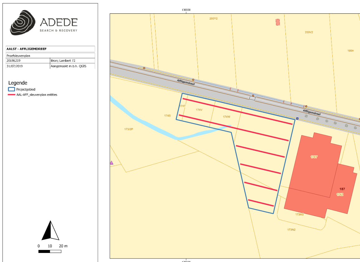
Figuur 3. Sleuvenplan.
