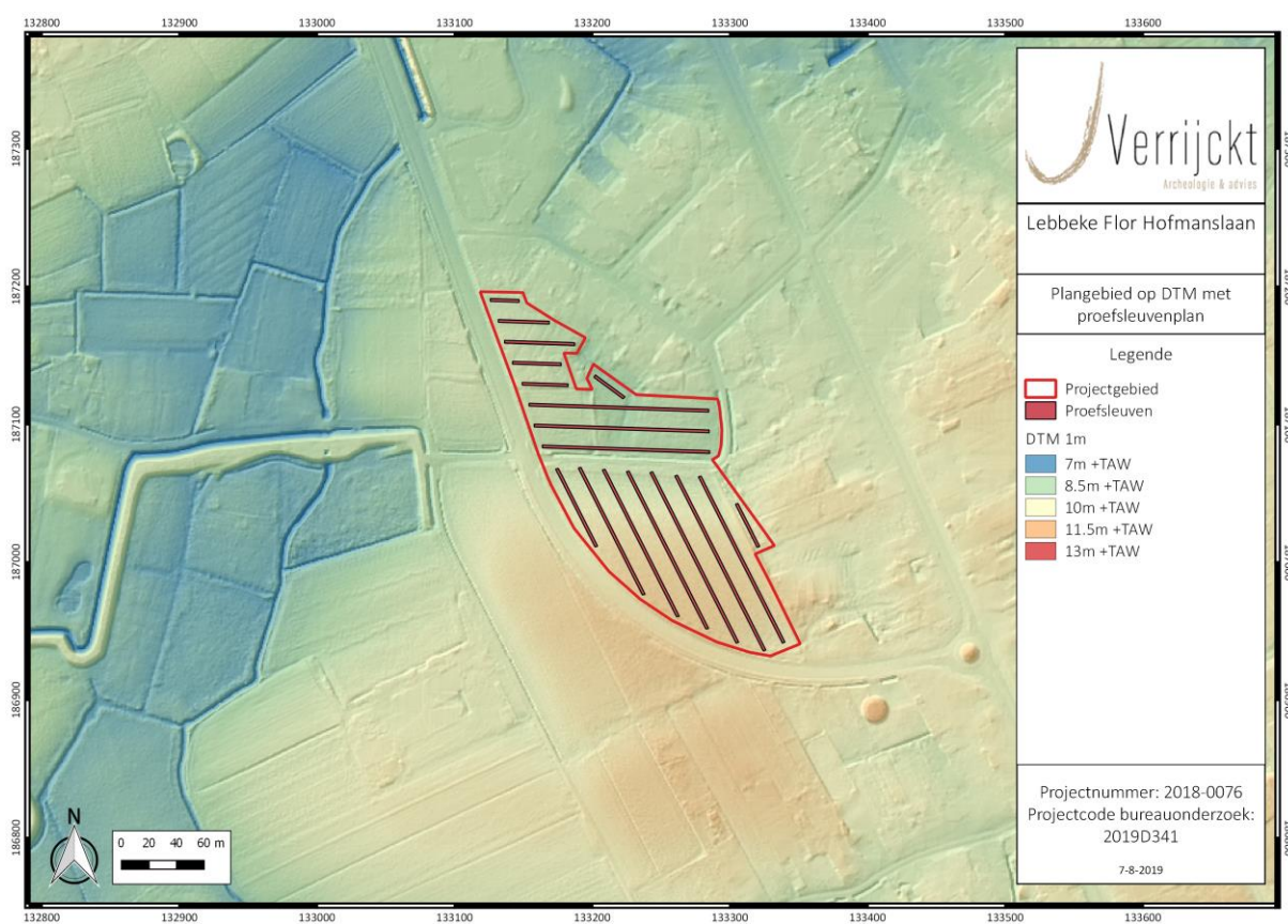
Figuur 4: Sleuvenplan op het DTM (Bron: AGIV)
