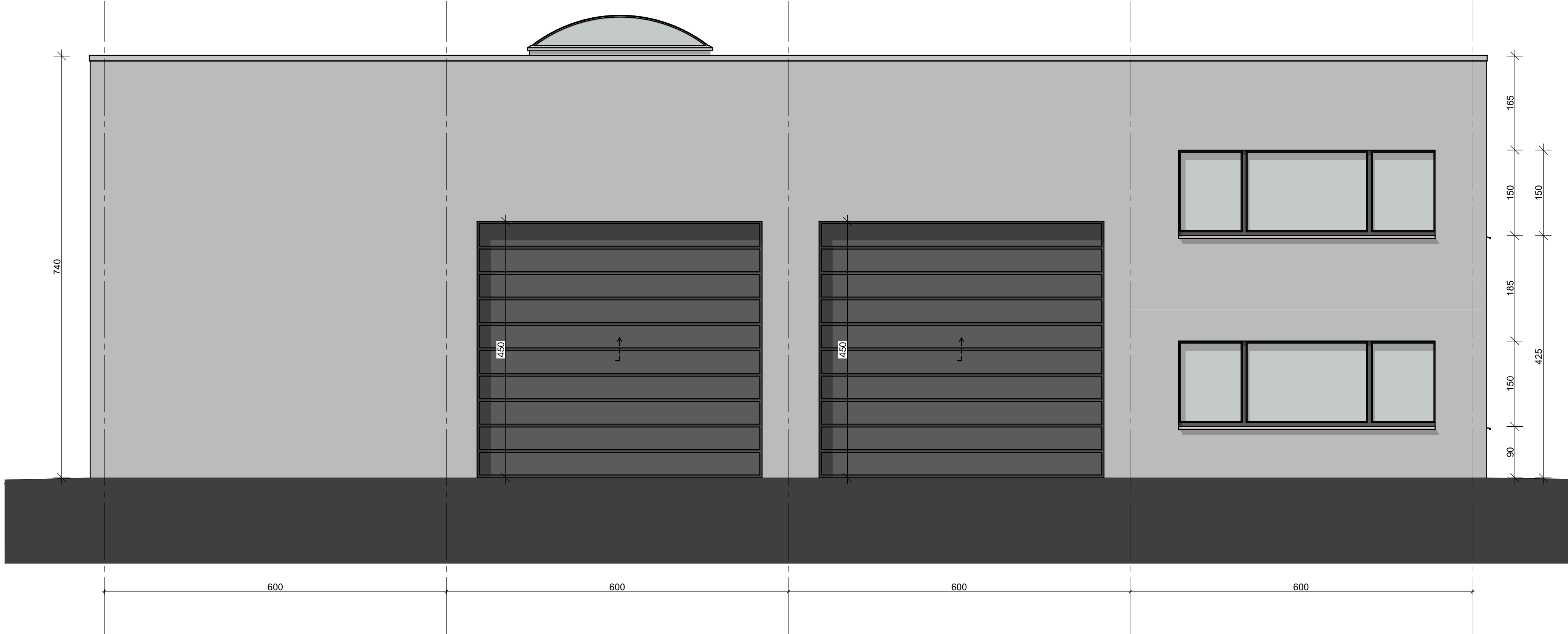
VOORGEVEL schaal 1/50
