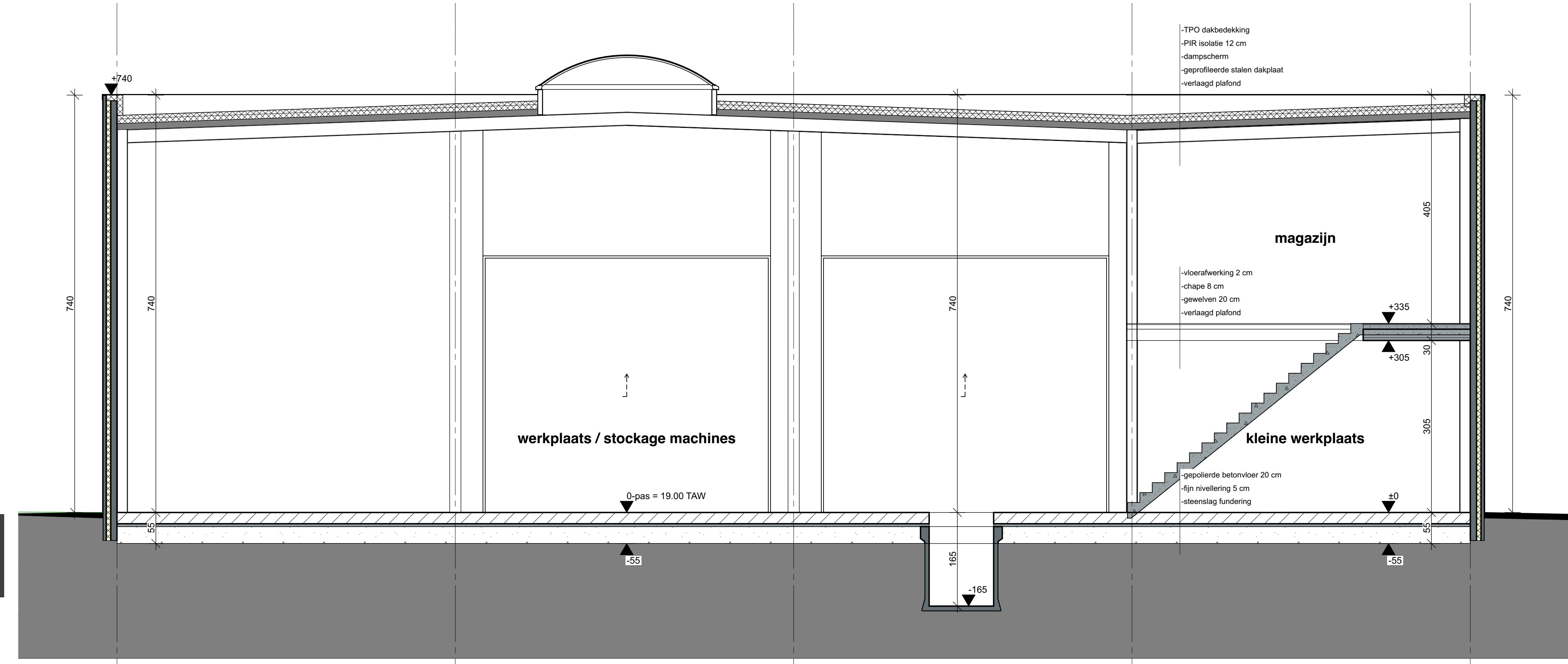
DOORSNEDE 2-2 schaal 1/50
