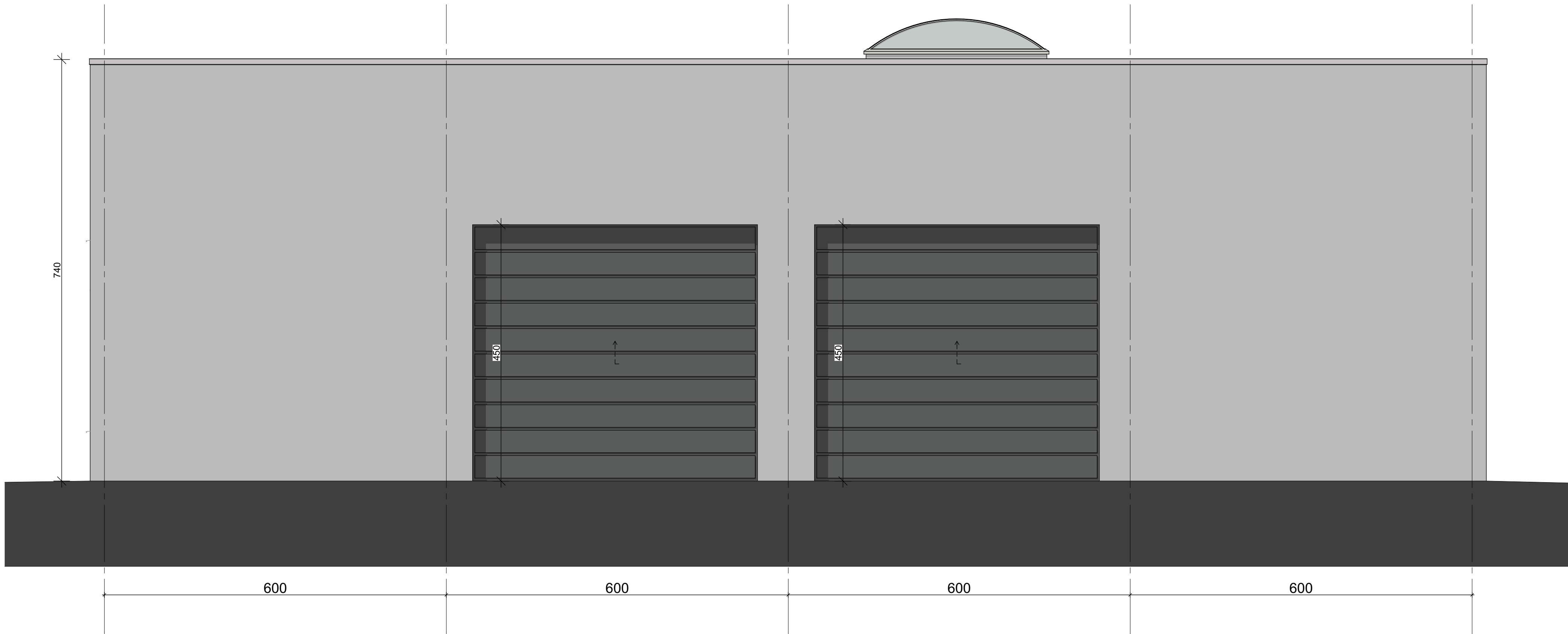
ACHTERGEVEL schaal 1/50
