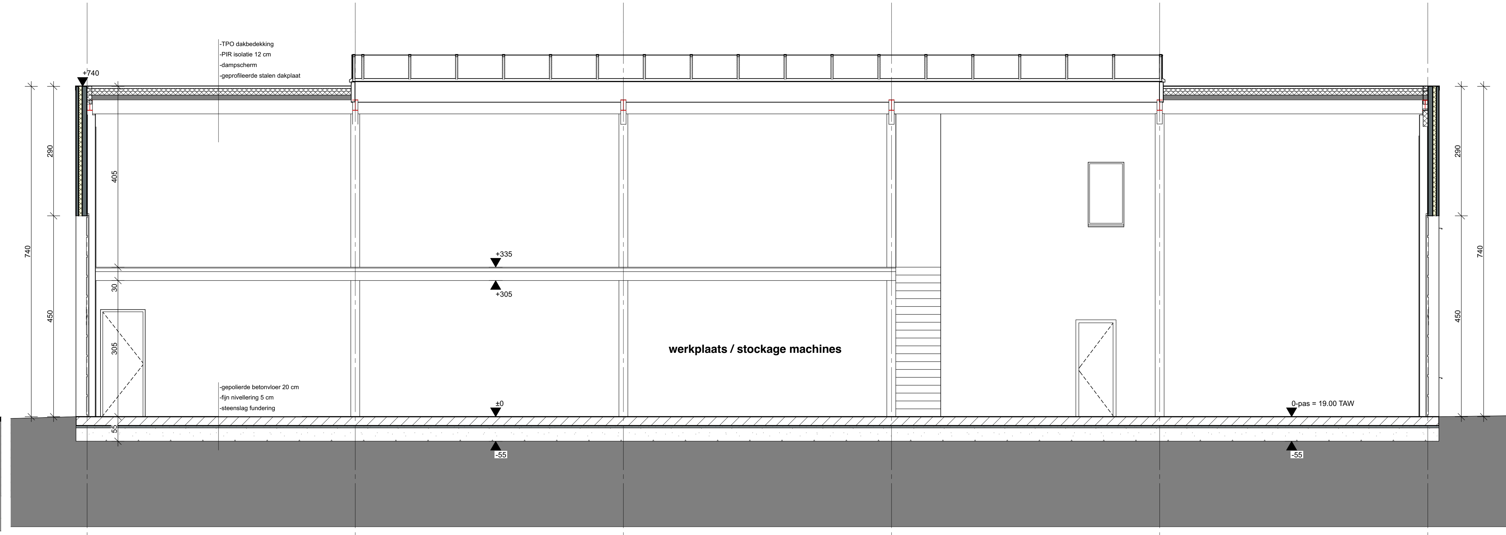
DOORSNEDE 5-5 schaal 1/50
