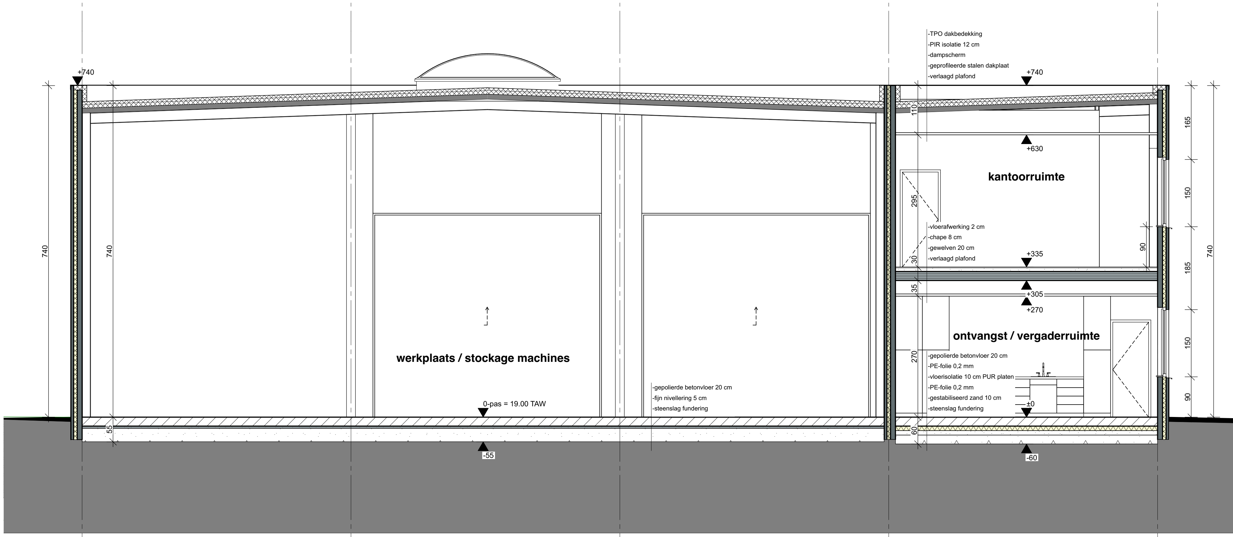
DOORSNEDE 1-1 schaal 1/50
