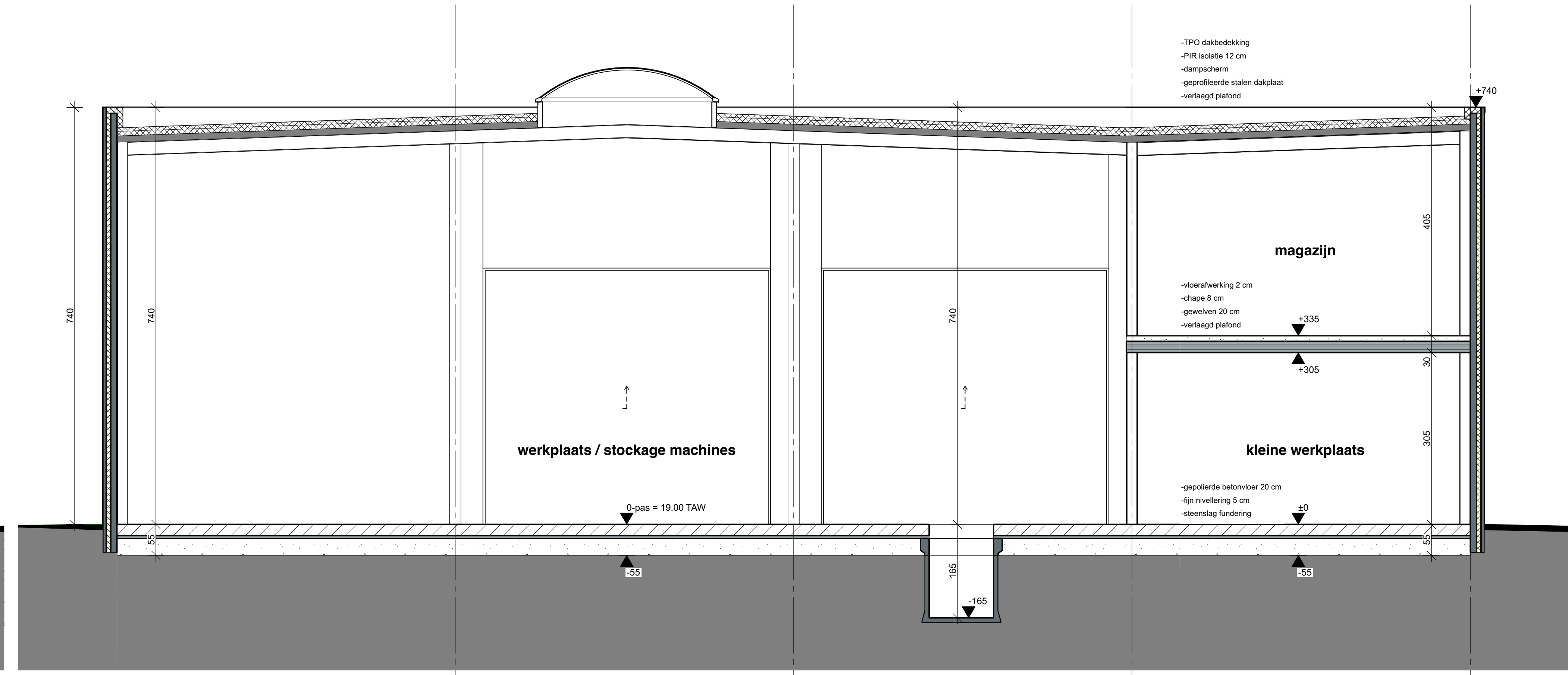
DOORSNEDE 3-3 schaal 1/50
