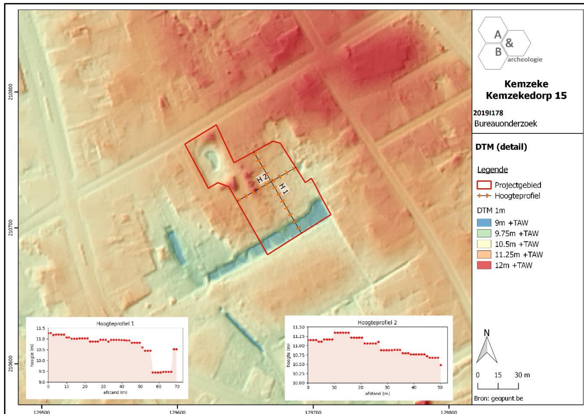
Figuur 15 Detailopname van het Digitaal Hoogtemodel met de twee hoogteprofielen; de gracht aan de zuidelijke grens is duidelijk waarneembaar, net als de vijver aan de straatzijde (bron: AGIV).
