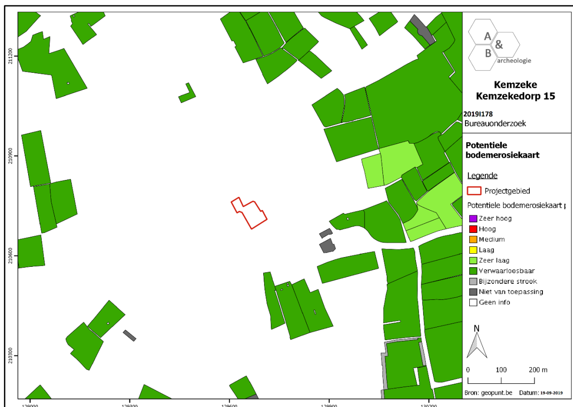
Figuur 16 Zicht op de Potentiële bodemerisiekkaart (bron: geopunt.be).
