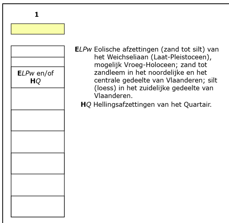
Figuur 21 Uitleg bij de Quartair Geologische Kaart; type 1 (bron: geopunt.be ).
