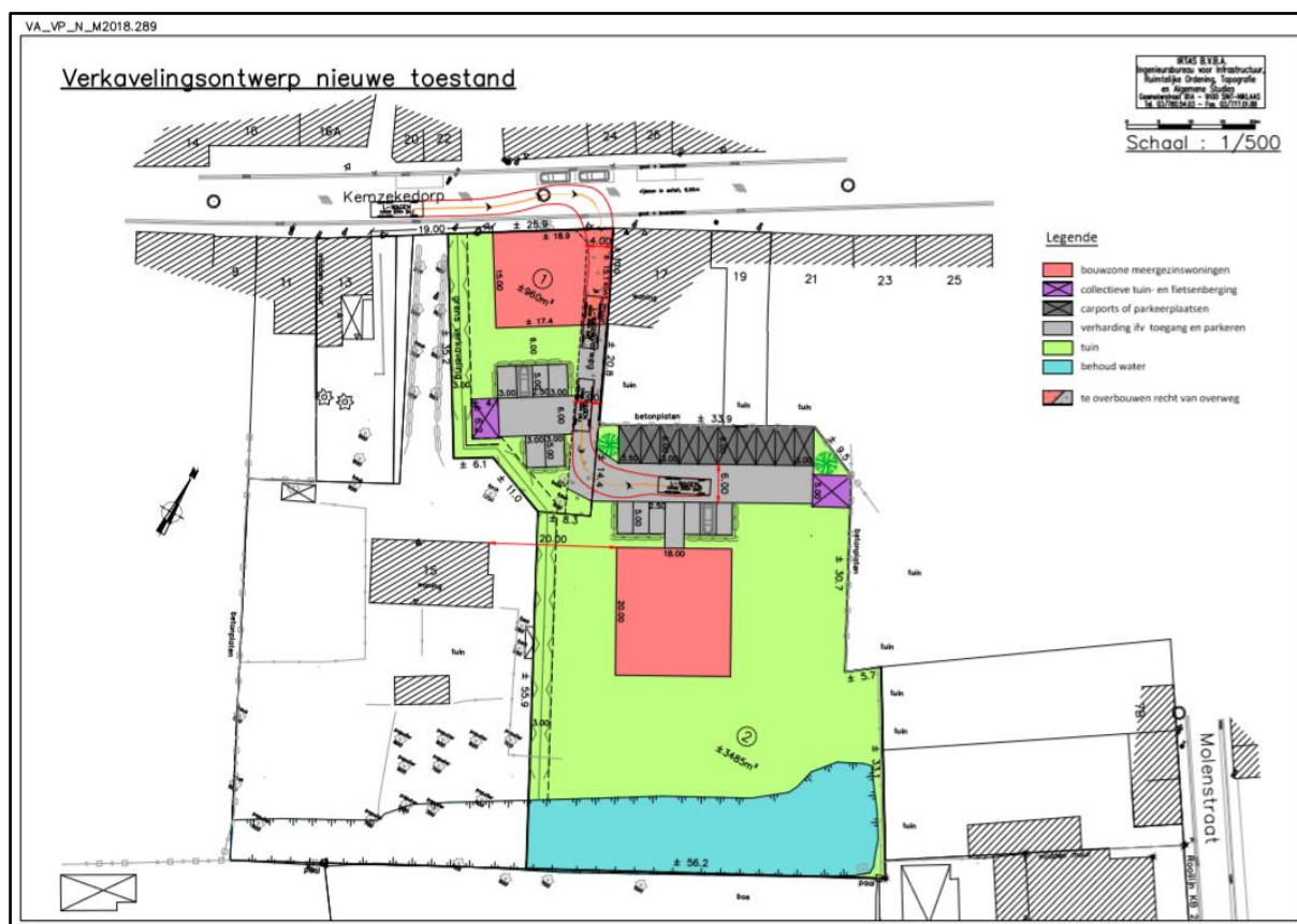
Figuur 9 Uitsnede uit het verkavelingsplan met inrit aanwijzing (bron: initiatiefnemer).
