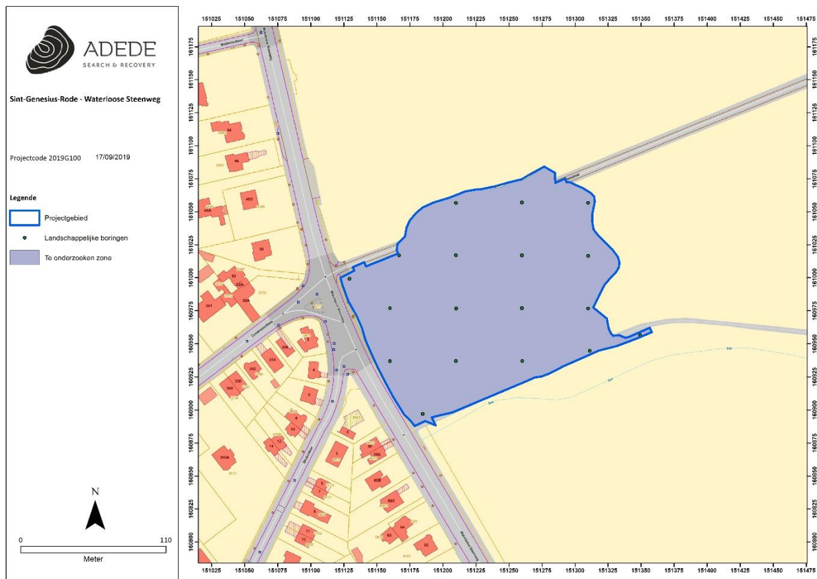
Figuur 2. Boorplan
