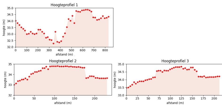
Figuur 14: Hoogteprofielen
