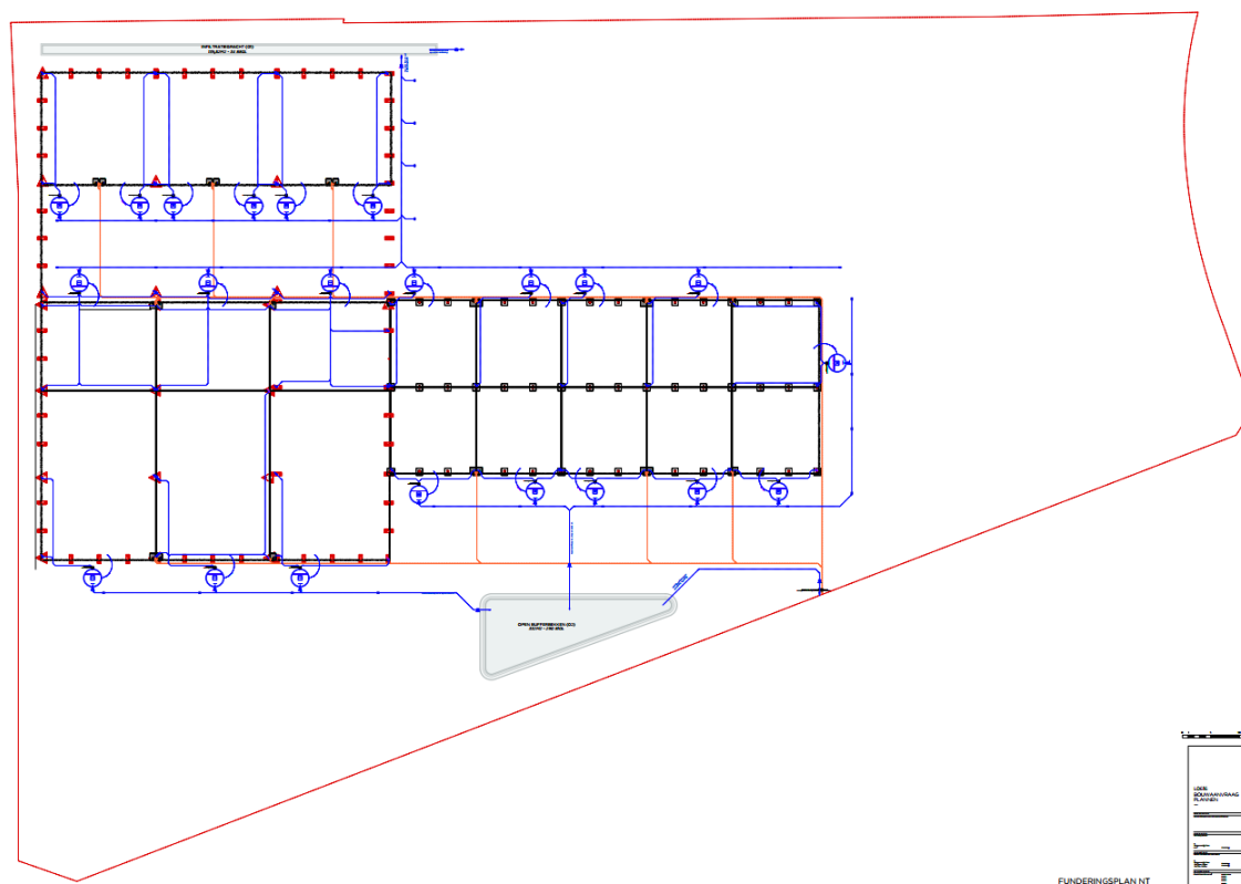
Figuur 8: Plangebied met weergave van toekomstige inplanting van de riolering en bufferbekken/gracht 11
