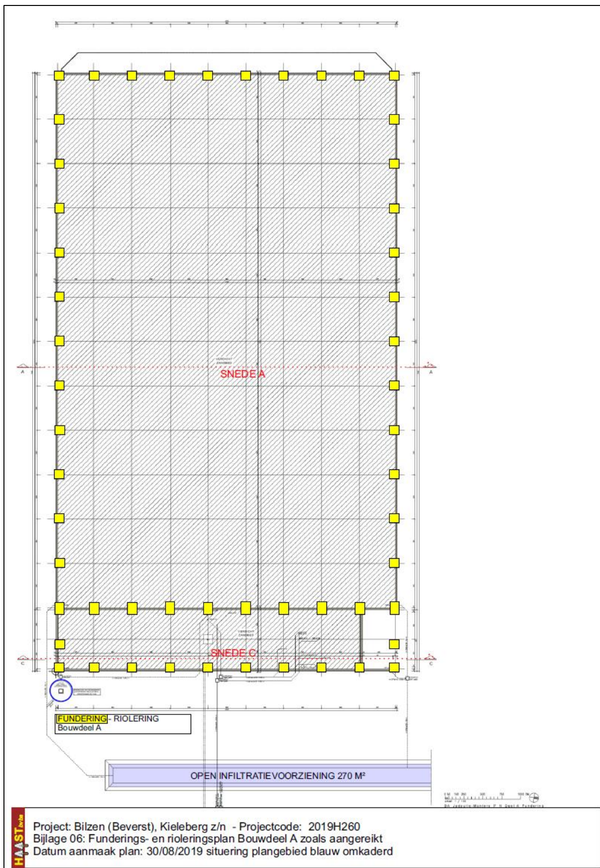
Fig. 8: funderings- en rioleringsplan bouwdeel A (productiehal en kantoren, sanitair, kleedruimten)
