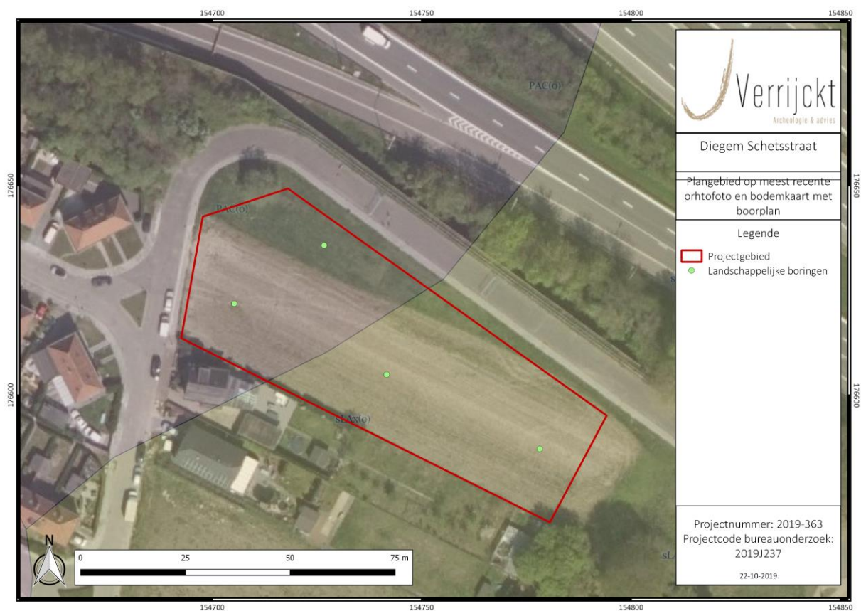
Figuur 3: Boorplan op meest recente orthofoto met bodemkaart als overlay (Bron: Geopunt)
