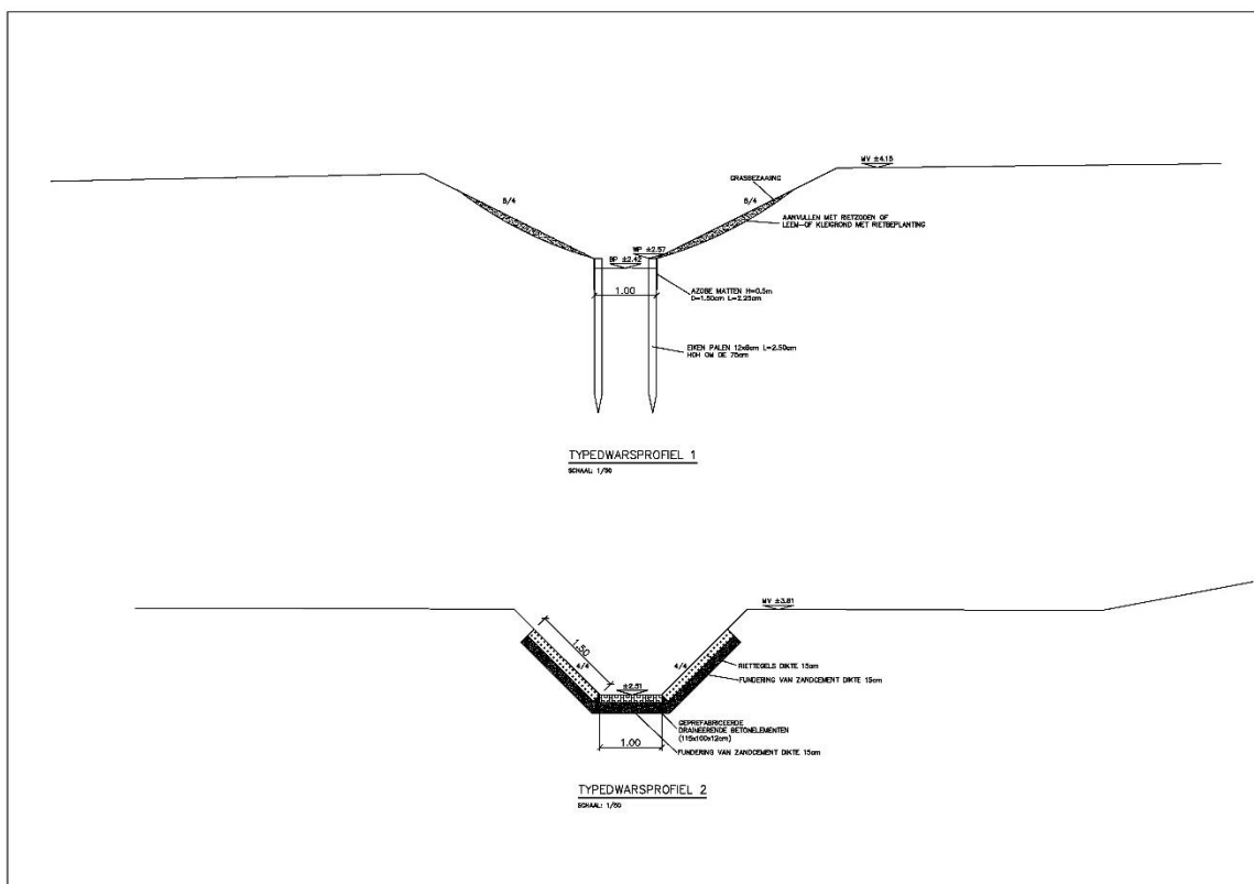
Figuur 6: Dwarsprofiel van de geplande gracht (cfr. Bijlage 2). 8
