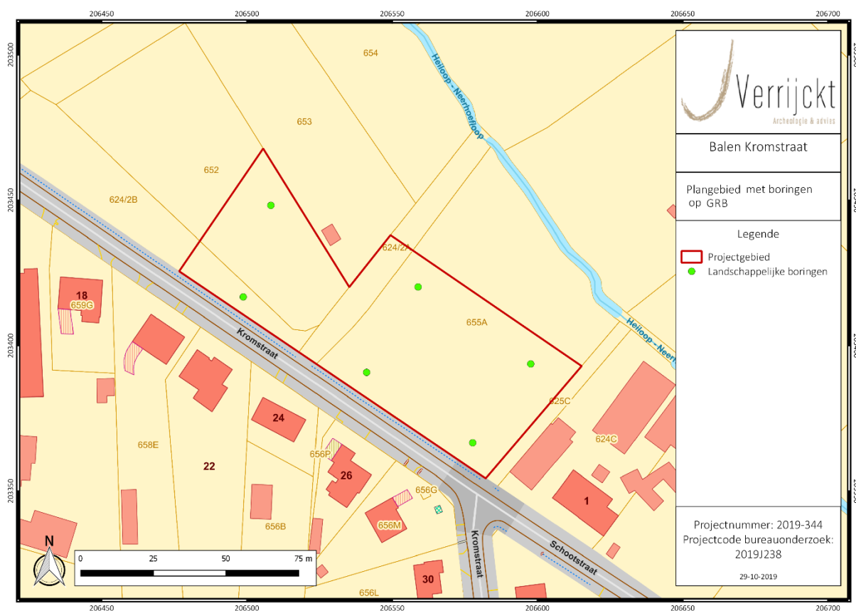
Figuur 2: Inplanting landschappelijke boringen op GRB 3
