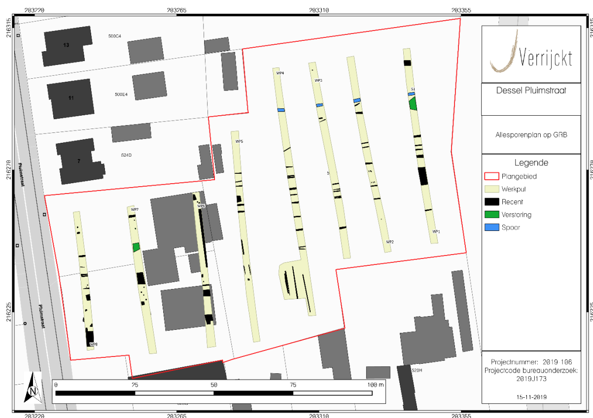
Figuur 1: Syntheseplan
