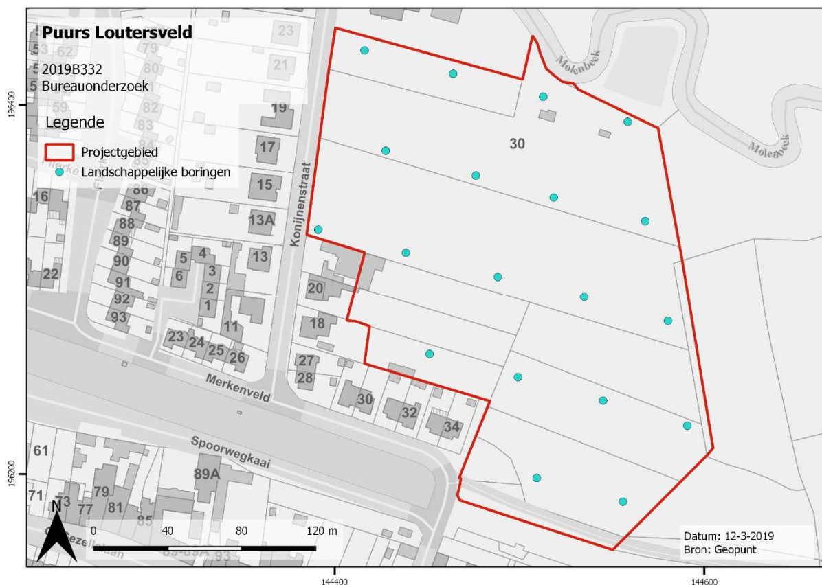
Figuur 2 Voorstel landschappelijke boringen. (bron: geopunt)
