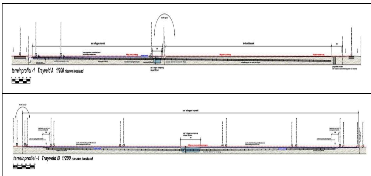
Figuur 8b. Snedes van de nieuwe trayvelden (boven: A; onder: B).
