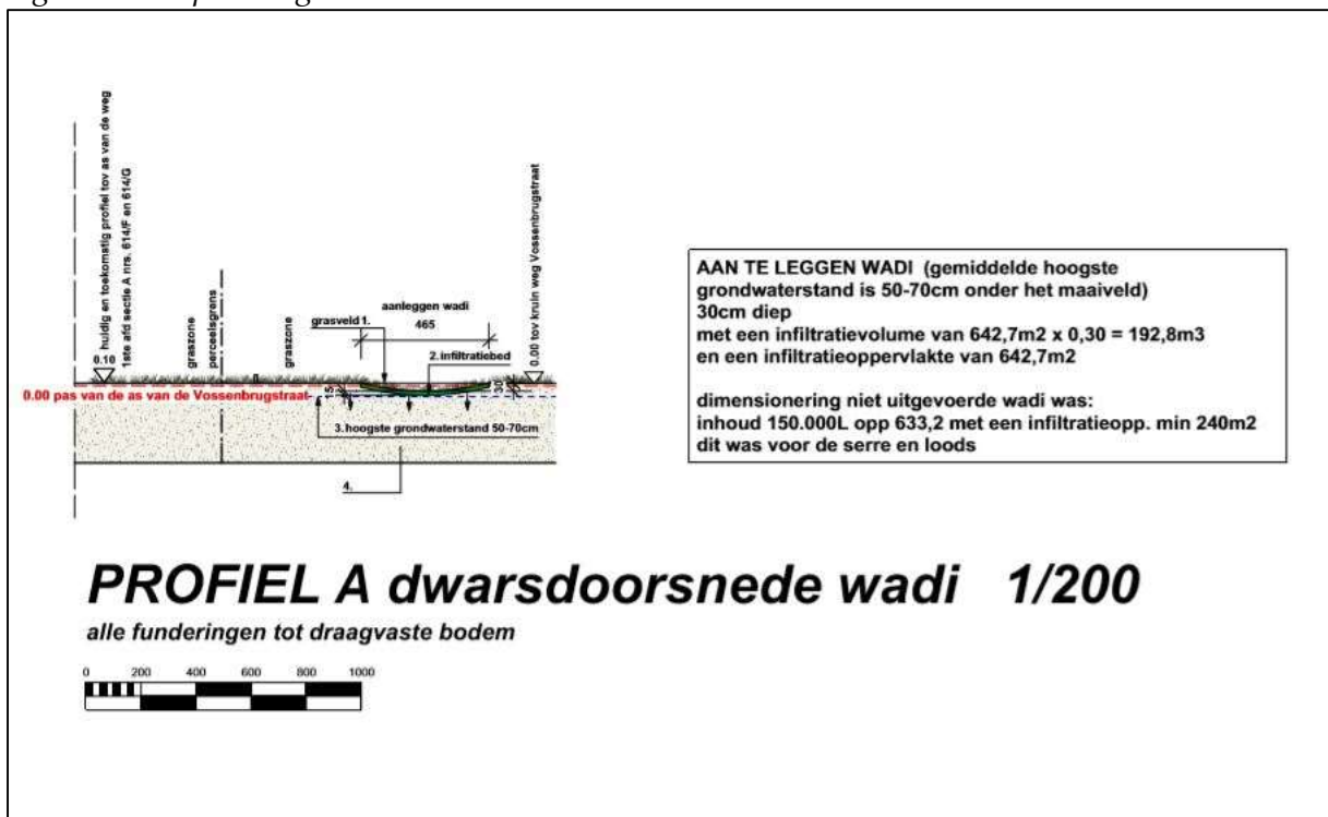
Figuur 9b. Doorsnede nieuwe wadi.
