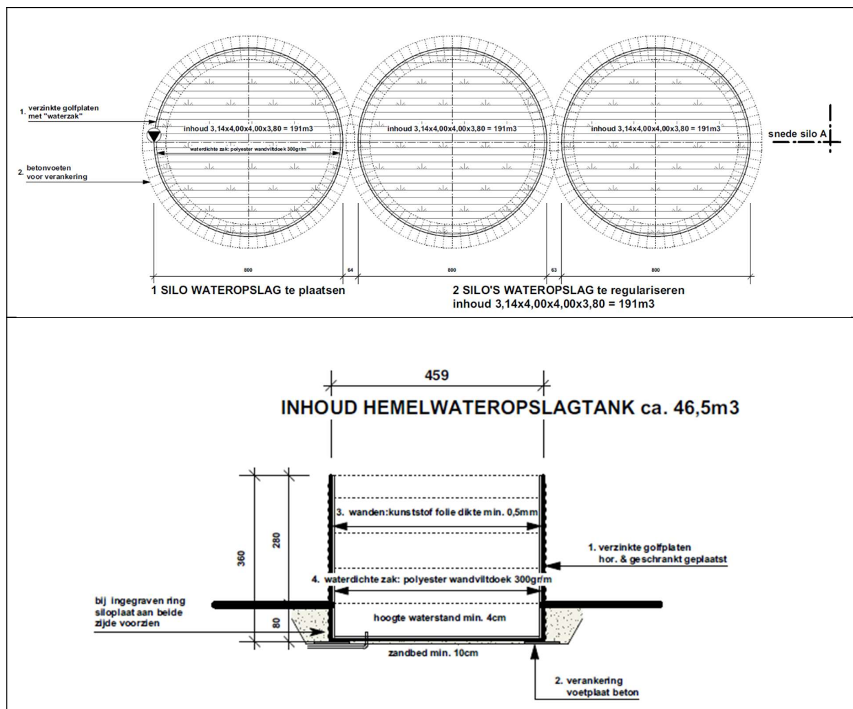
Figuur 10f. Grondplan en sneede silo's.
