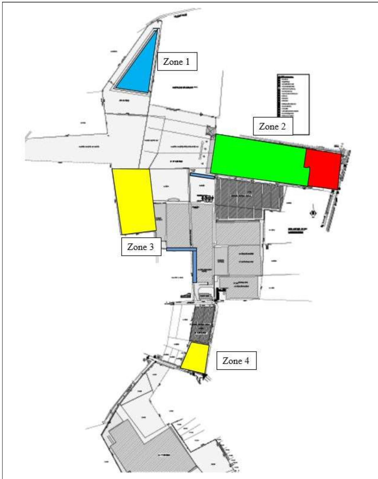
Figuur 6a. Interpretatietekening van het inplantingsplan van de nieuwe toestand: trayvelden (geel), tuinbouwserre (groen), tuinbouwloods (rood), waterbekkens en gracht (blauw).
