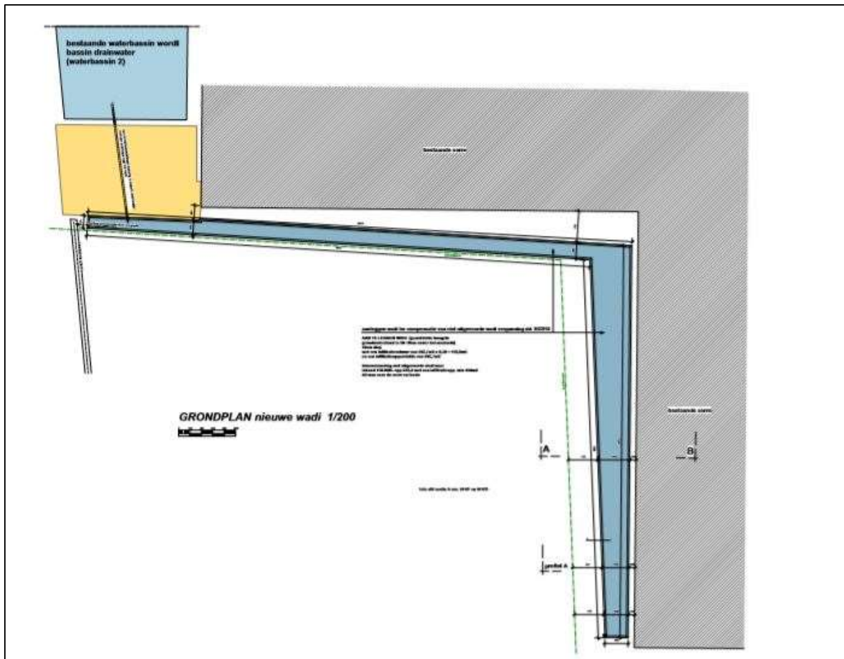
Figuur 9a. Inplanting van de nieuwe wadi.
