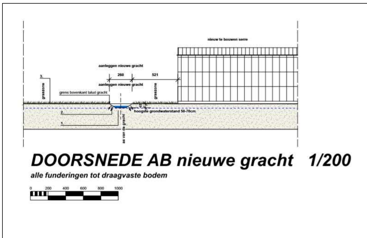
Figuur 10e. Doorsnede van de nieuwe gracht.
