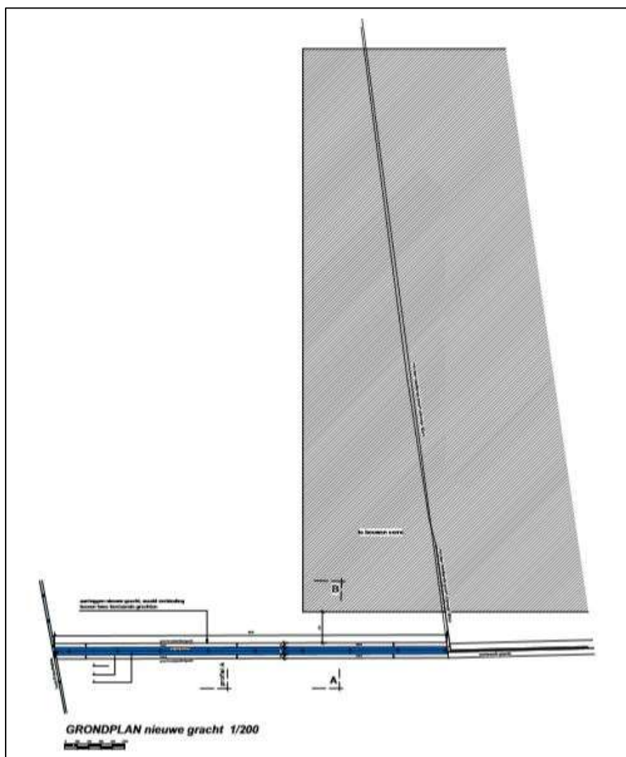
Figuur 10c. Grondplan van de nieuwe gracht
