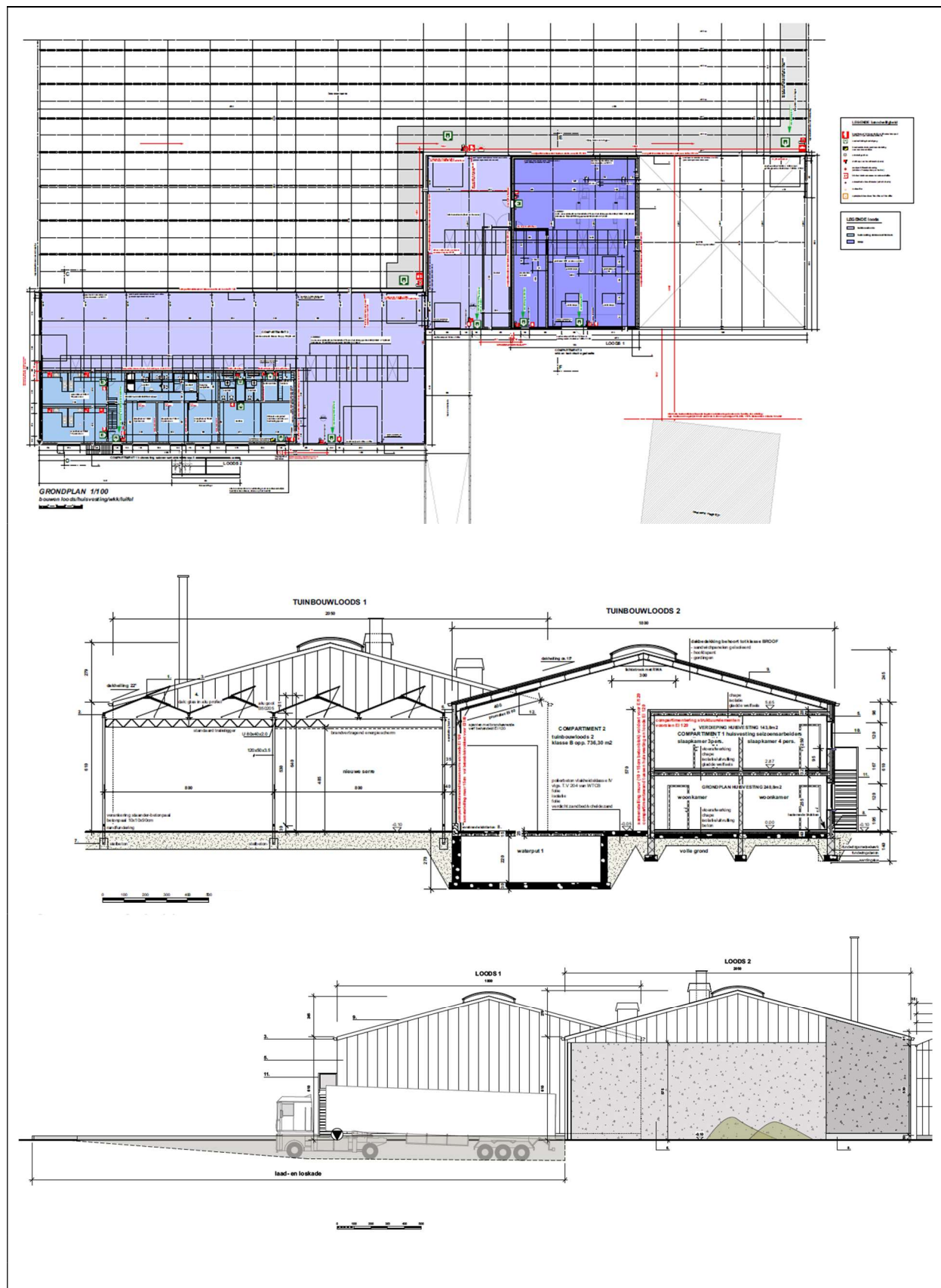
Figuur 10d. Inplantingsplan en snede van de tuinbouwloodsen.
