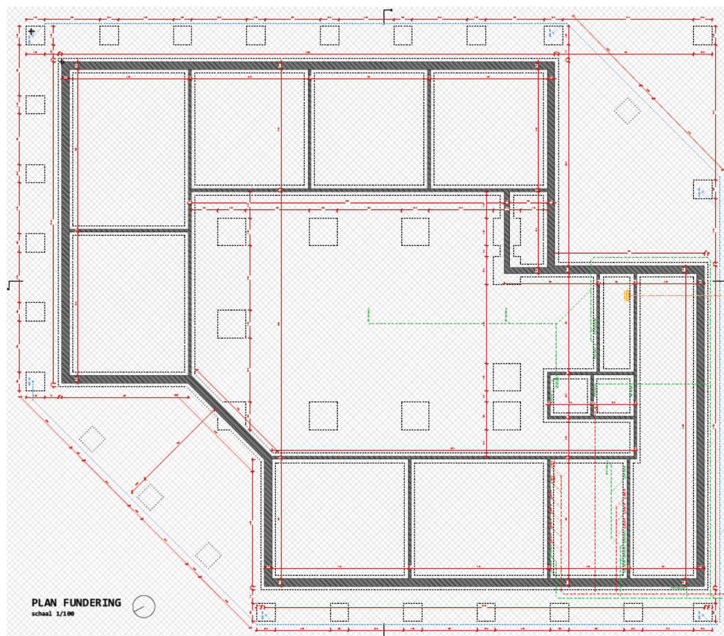
Afb. 4. Plan van de fundering en de riolering.
