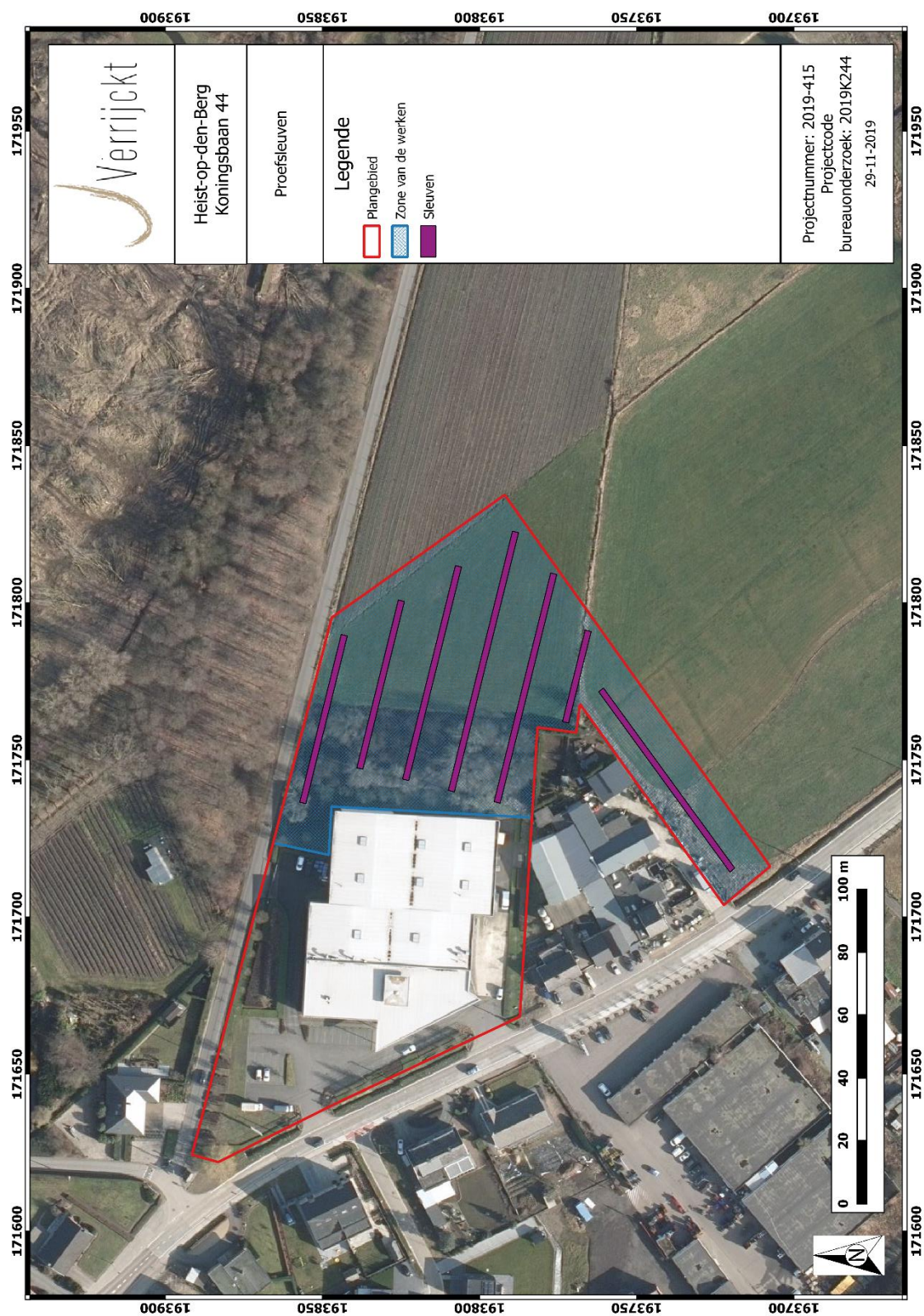
Figuur 4: Sleuvenplan
