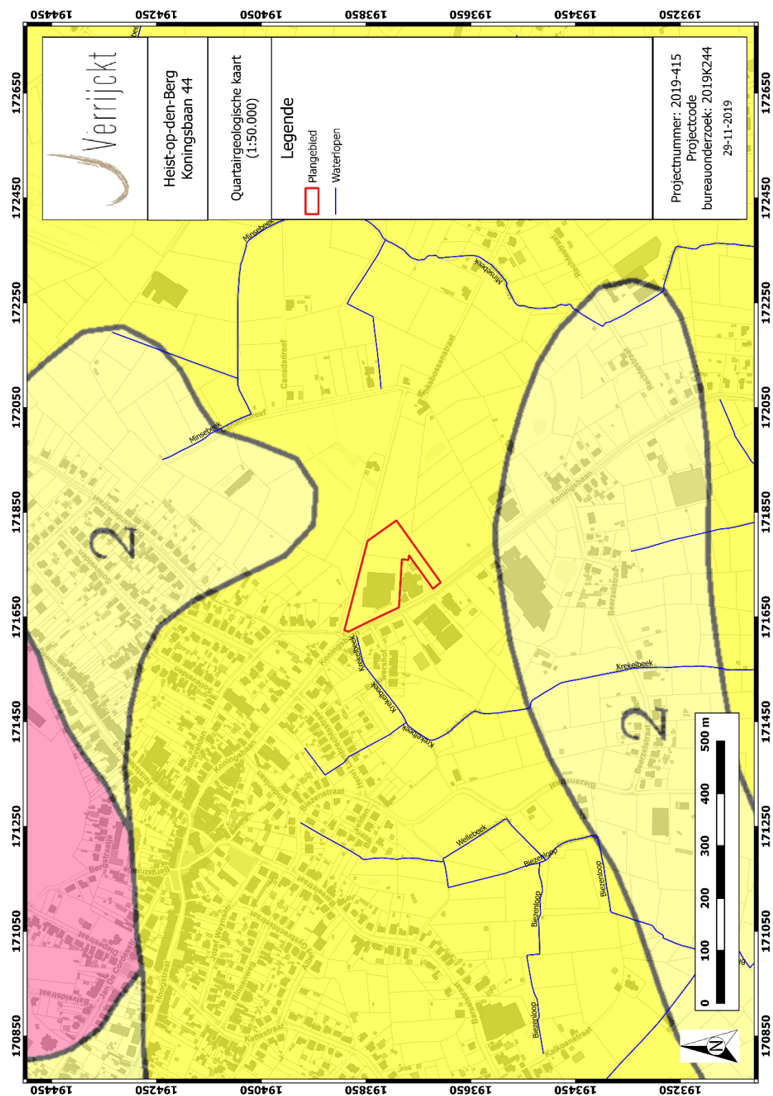
Figuur 16: Plangebied op de Quartairegeologische kaart 1:50.000 20
