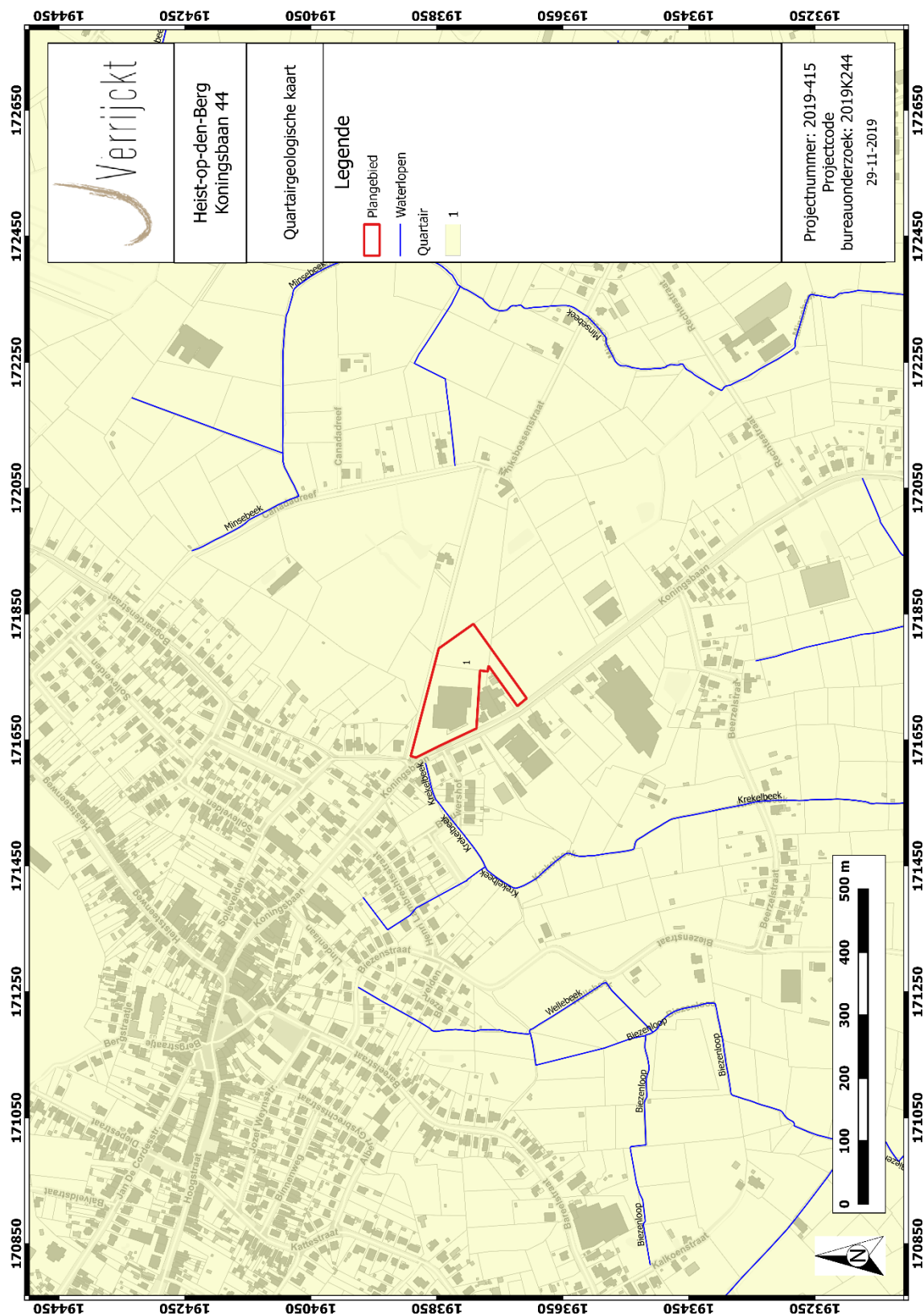
Figuur 14: Plangebied op de Quartaairgeologische kaart 1:200.000 18
