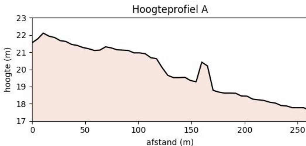
Figuur 11: Hoogteprofiel A (west-oost) 15
