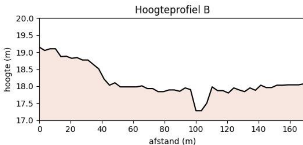
Figuur 12: Hoogteprofiel B (zuidwest-noordoost) 16
