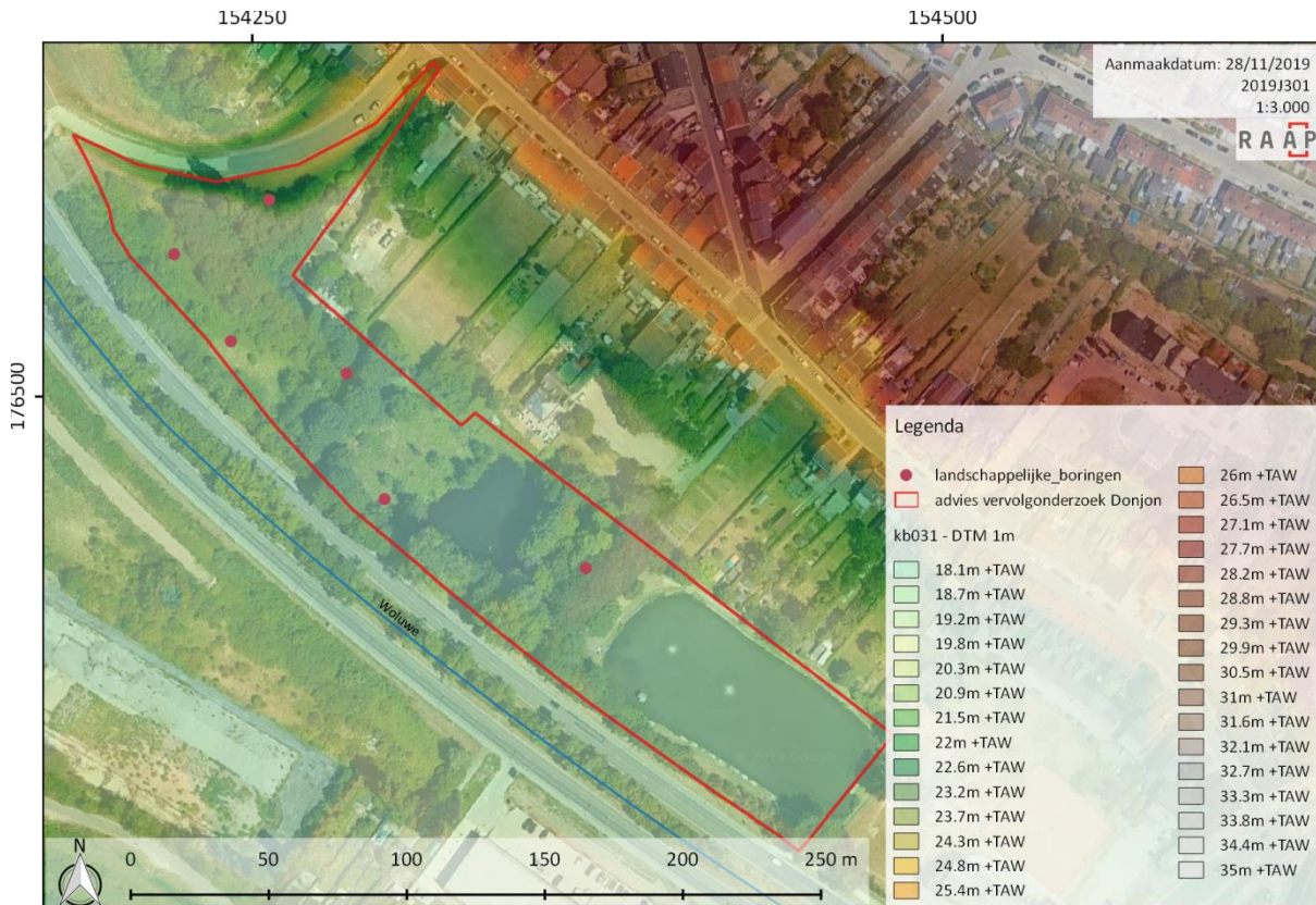
Figuur 10 Voorstel voor landschappelijke boringen binnen het deelgebied Donjon (bron: Geopunt, 2018; AGIV, 2019b)
