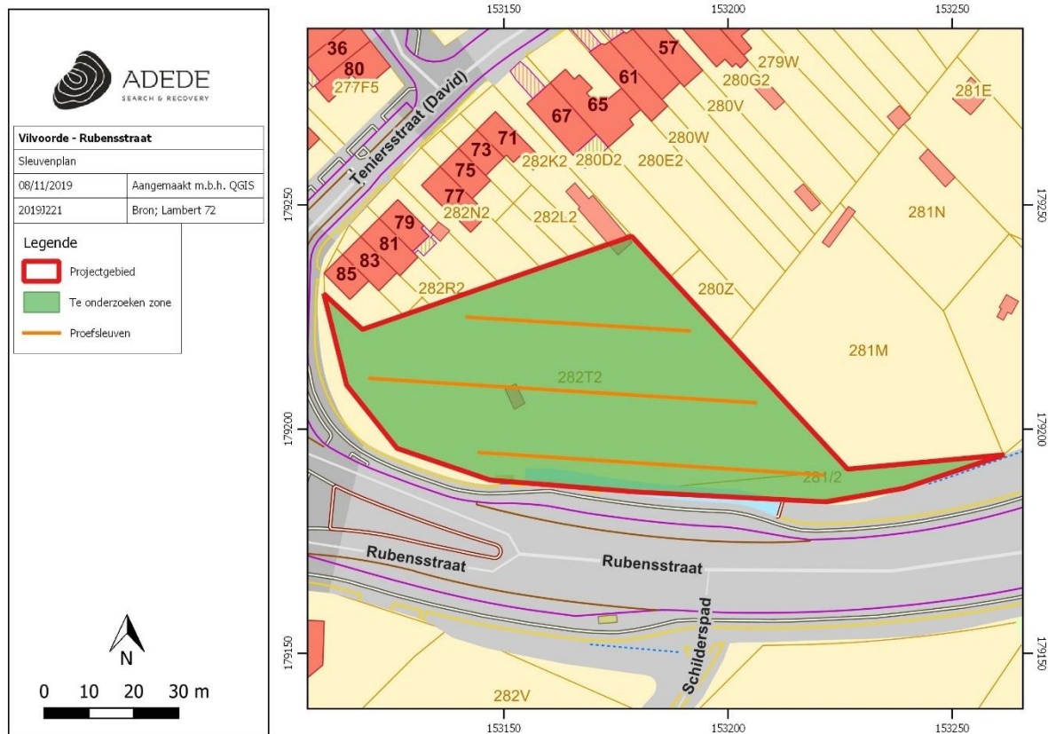
Figuur 3. Sleuvenplan
