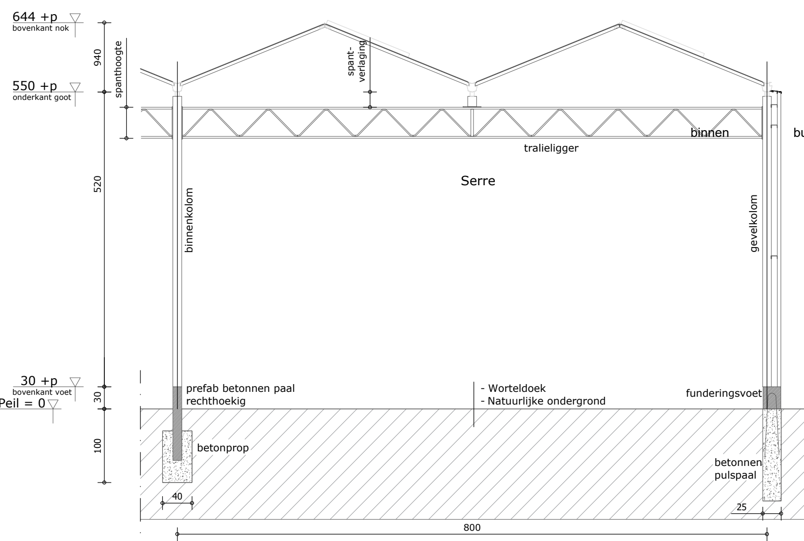
- principe serereconstructie 1/50 -
