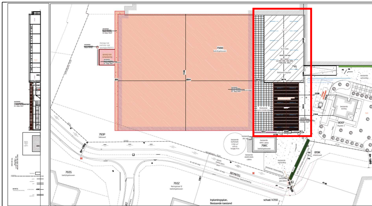
Figuur 3. Inplantingsplan detail. De rode kader geeft aan waarop figuur 4 slaat (funderingsplan).
