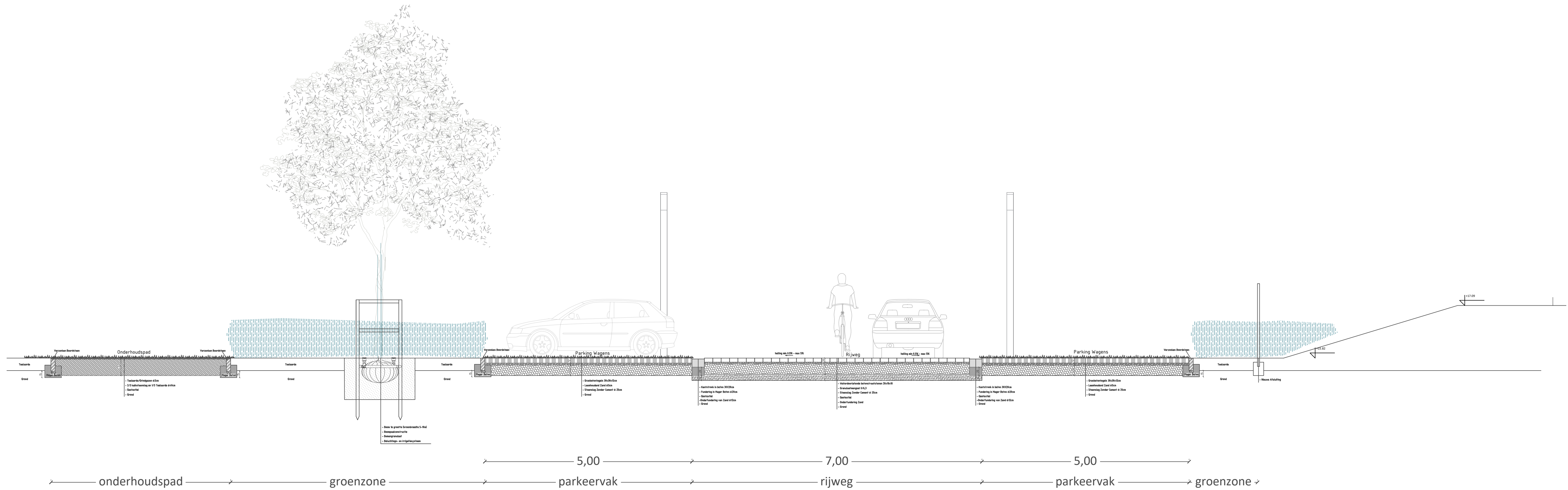
| PROFIEL BB' |
