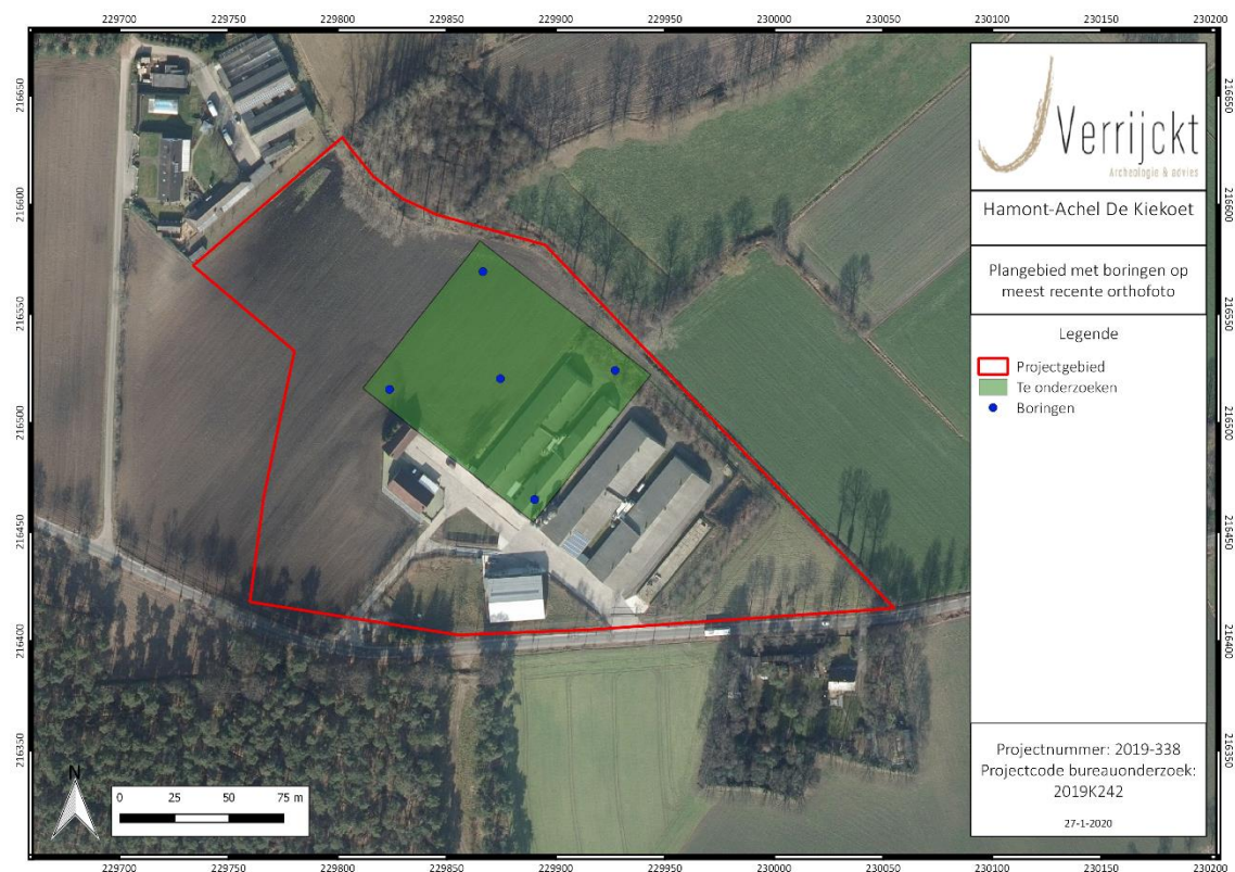
Figuur 3: Inplanting landschappelijke boringen op meest recente orthofoto 4
