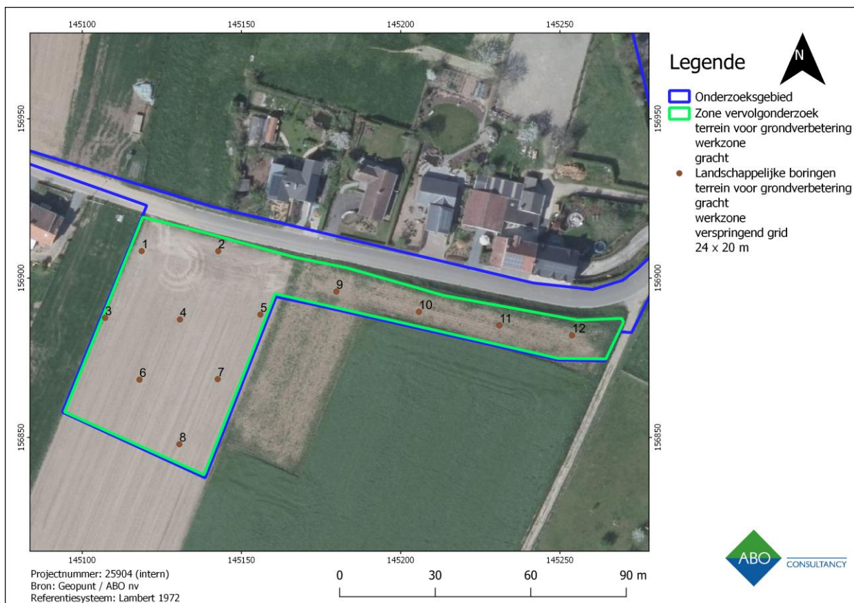
Figuur 5: Luchtfoto 2019 met aanduiding van de boorpunten voor het landschappelijk bodemonderzoek ter hoogte de zone voor de aanleg van het terrein voor grondverbetering, werkzone en gracht.
