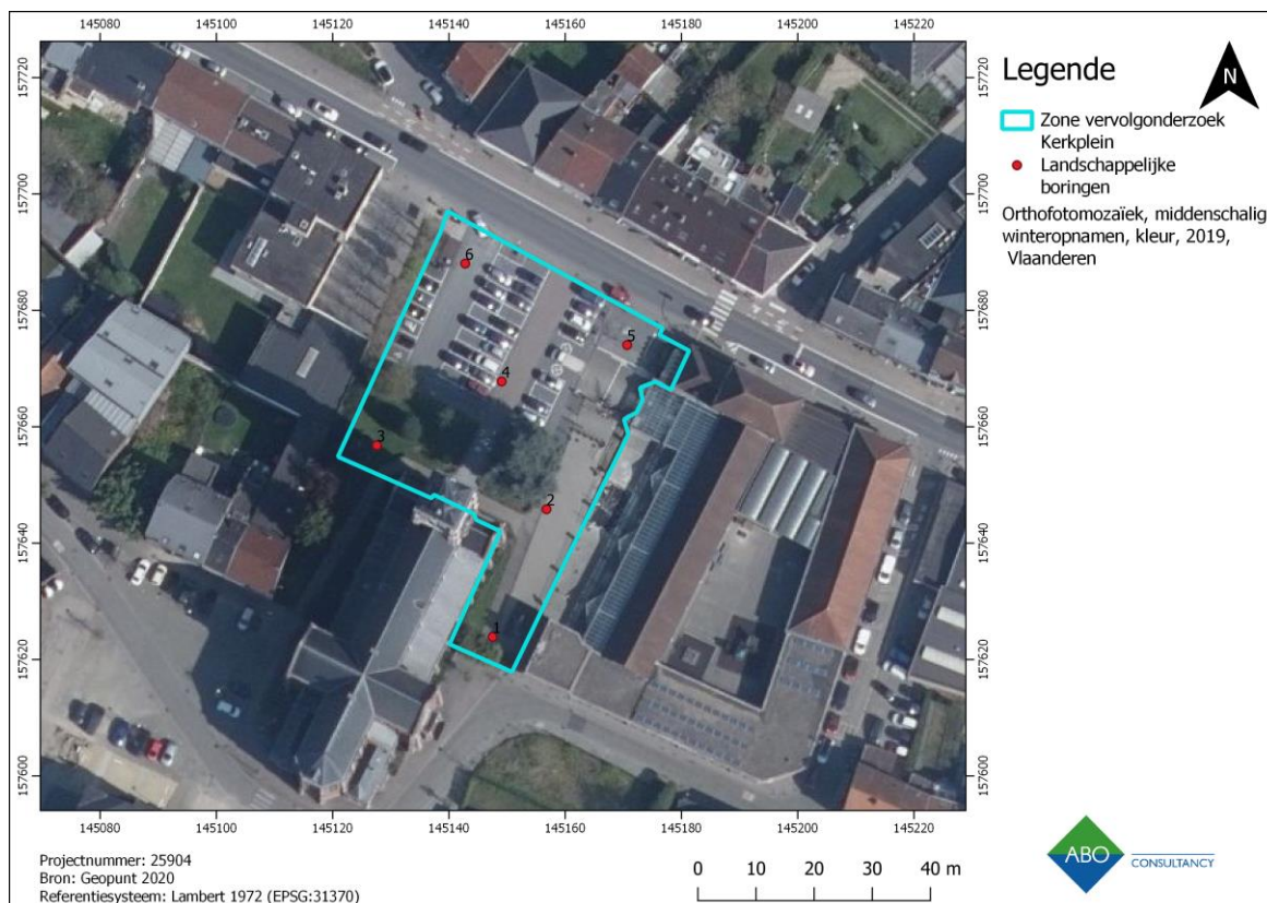
Figuur 7: Luchtfoto 2019 met aanduiding van de boorpunten voor het landschappelijk bodemonderzoek binnen het kerkplein.
