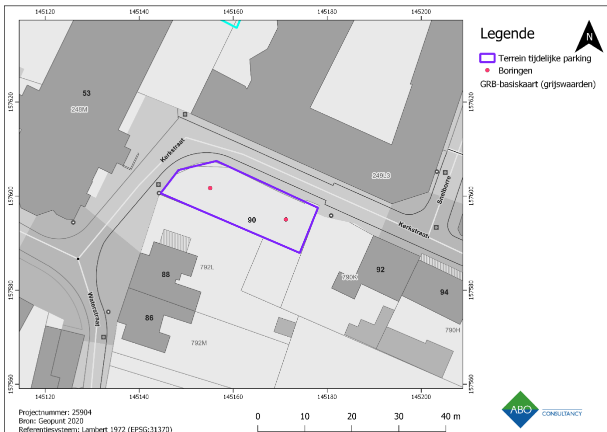
Figuur 10: GRB met aanduiding van de boorpunten voor het landschappelijk bodemonderzoek binnen het terrein voor tijdelijke parking.
