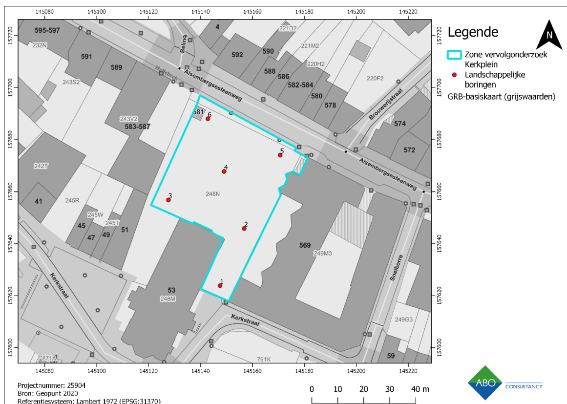
Figuur 8: GRB met aanduiding van de boorpunten voor het landschappelijk bodemonderzoek binnen het kerkplein.
