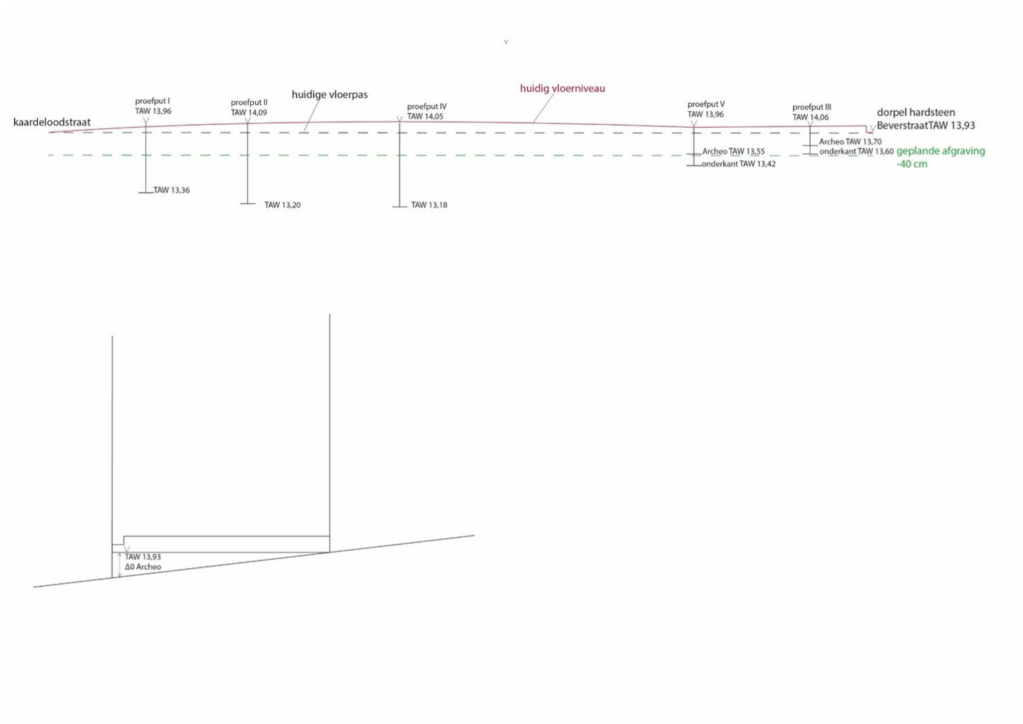
Figuur 47: Principeschets lengteprofiel en dwarsprofiel van het projectgebied met de absolute hoogtes van de proefputten (bron: SOLVA)
