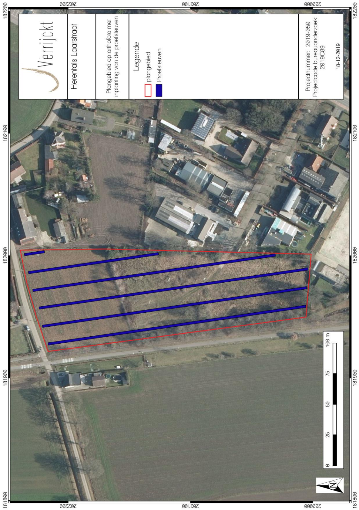
Figuur 3: Sleuvenplan
