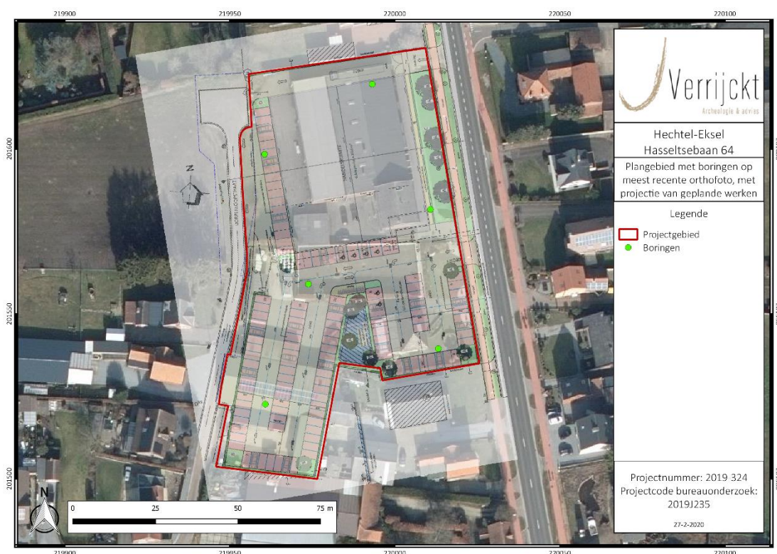
Figuur 4: Inplanting landschappelijke boringen met de geplande werken 5 op orthofoto 6
