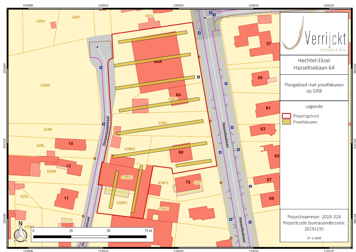
Figuur 5: Sleuvenplan op het GRB 12
