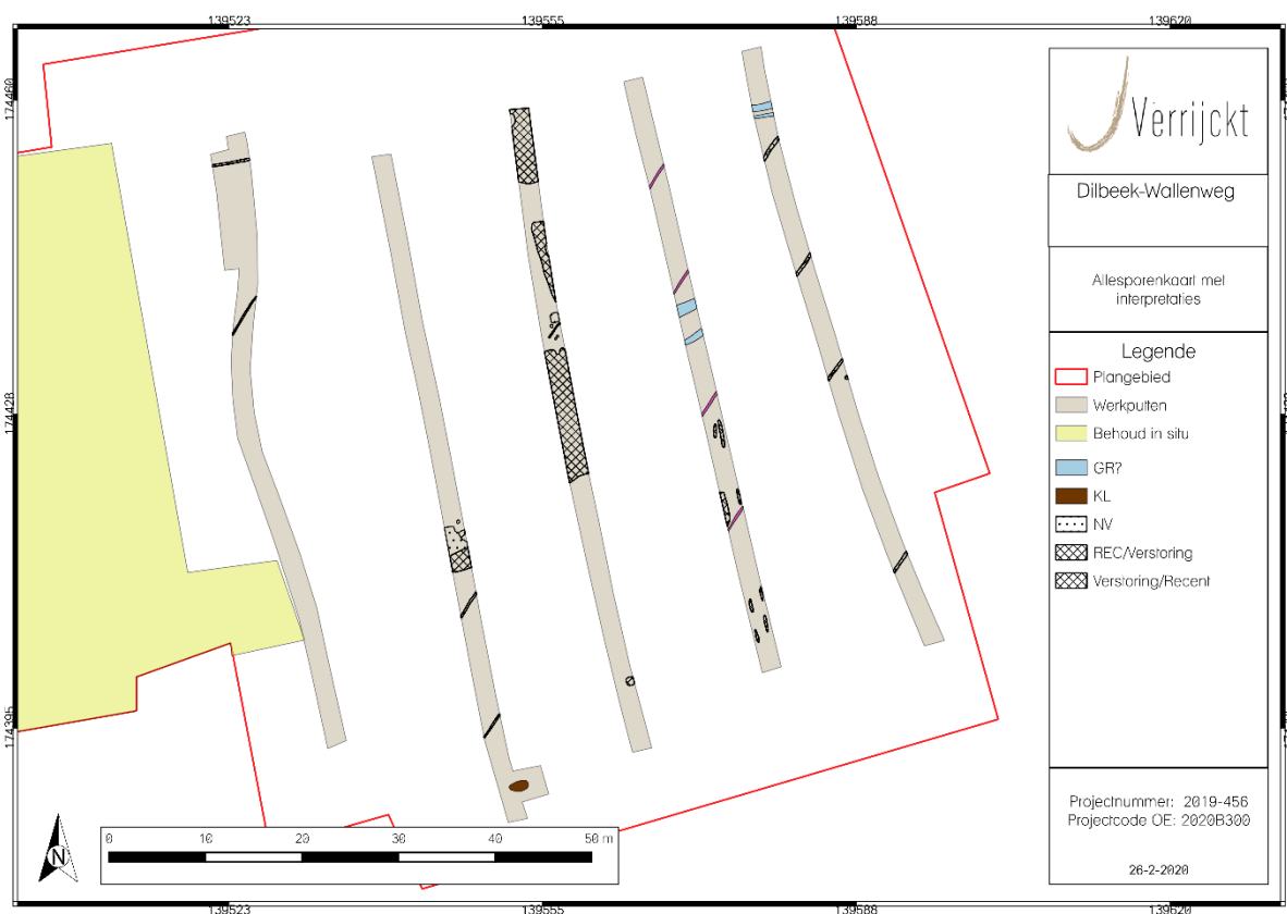
Figuur 1: Syntheseplan
