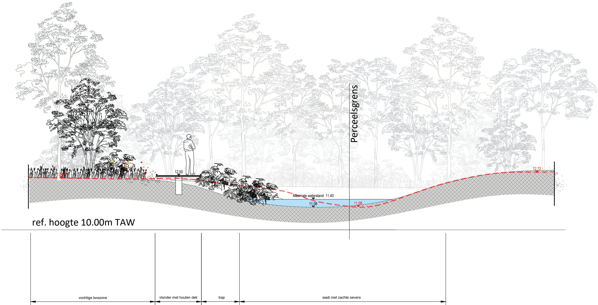
DOORSNEDE DD'
