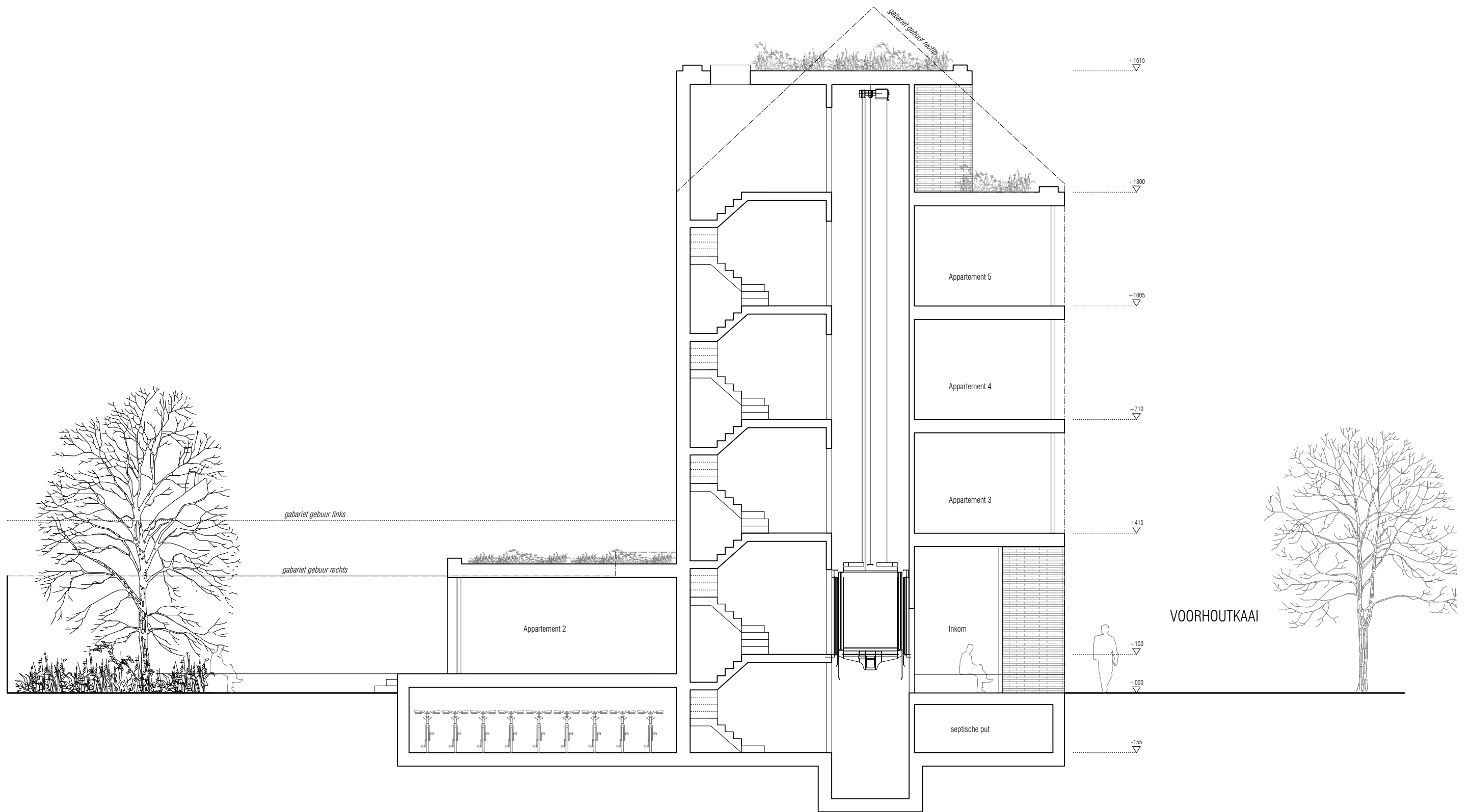
verticale snede AA' (schaal 1/100)
