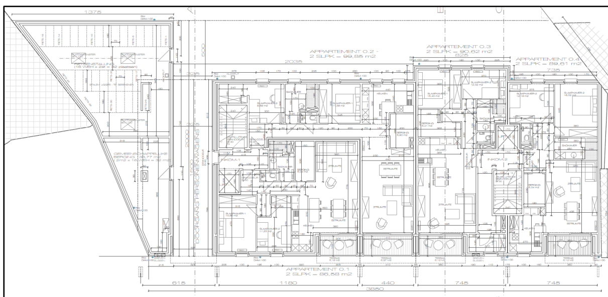
Figuur 6: Grondplan nieuwbouw appartementen 10
