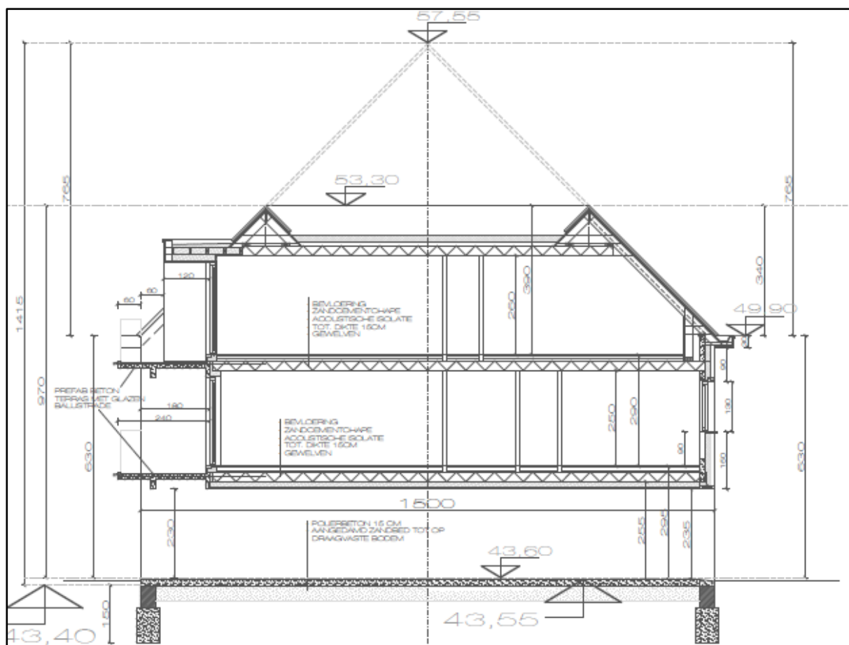
Figuur 8: Doorsnede AA nieuwbouw appartementen 12
