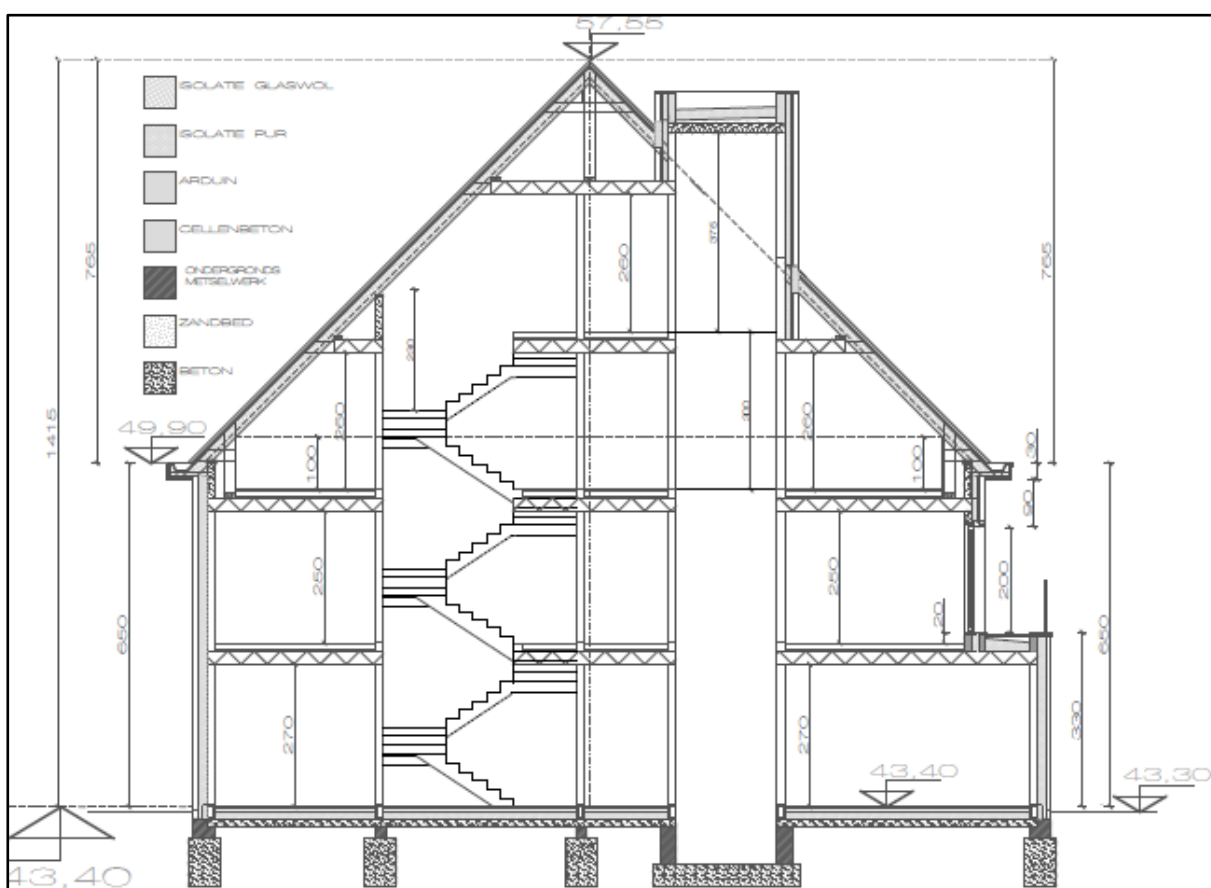
Figuur 7: Doorsnede CC nieuwbouw appartementen 11
