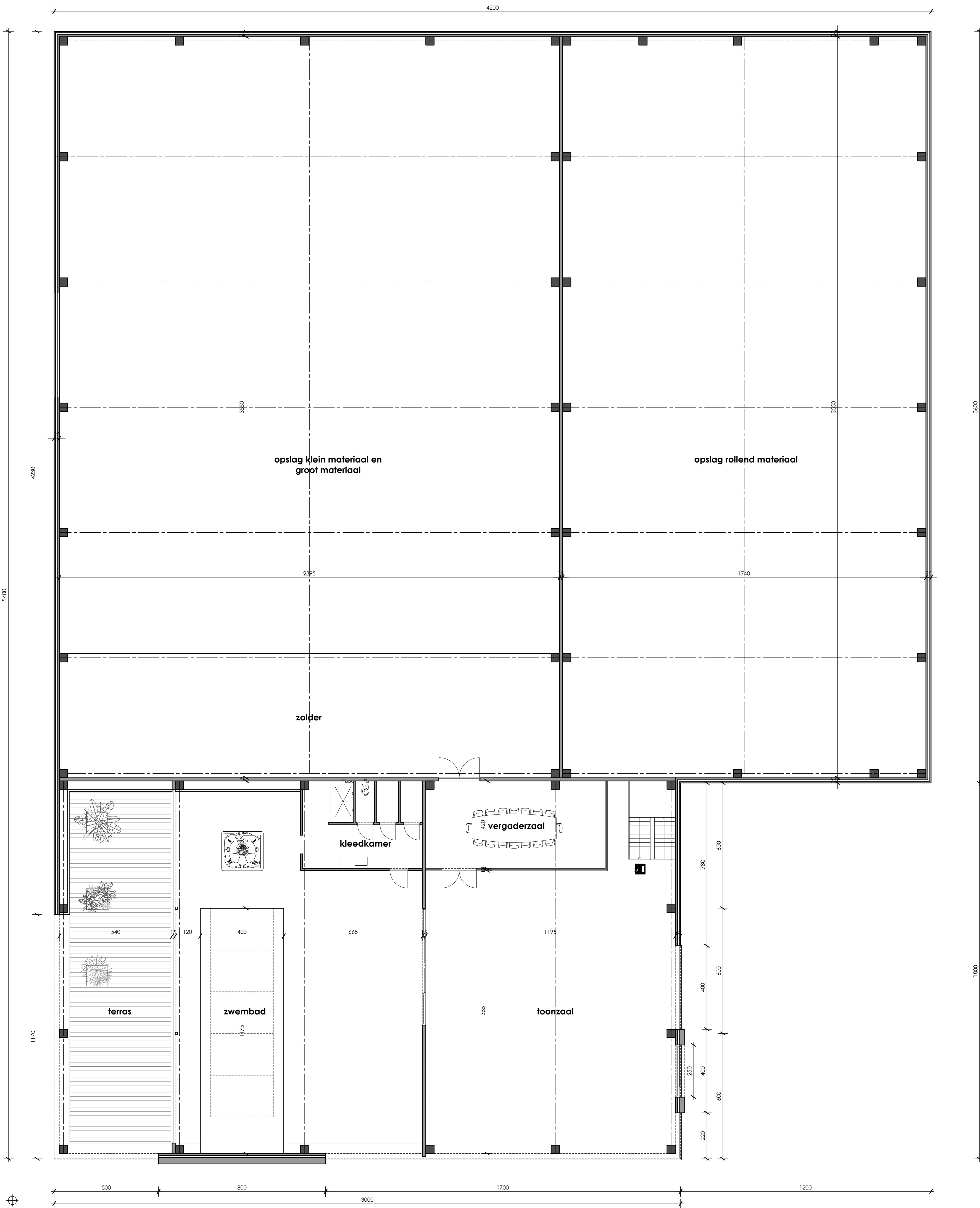
Verdieping 1/100
