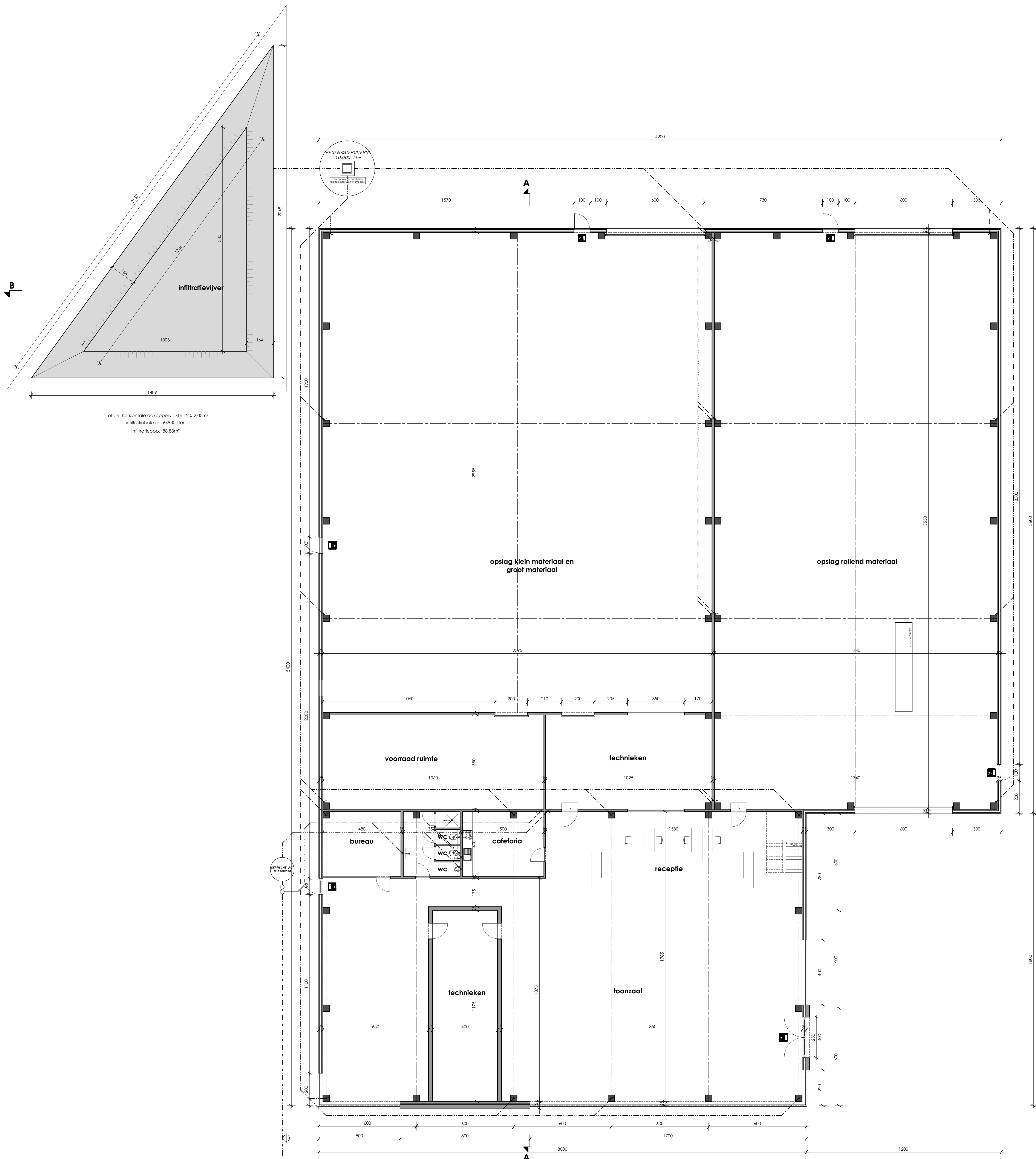
Funderings-, Rioleringsplan & Grondplan 1/100
