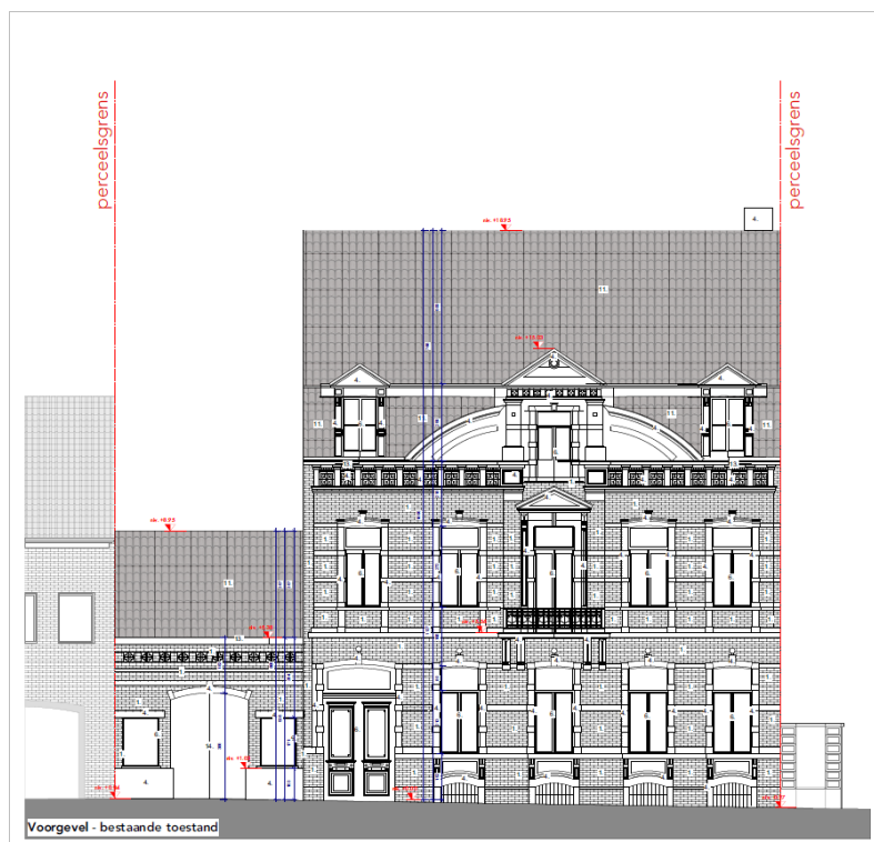
Figuur 5: Bestaande voorgevel (Drieskens & Dubois architecten cvba, 2020)
