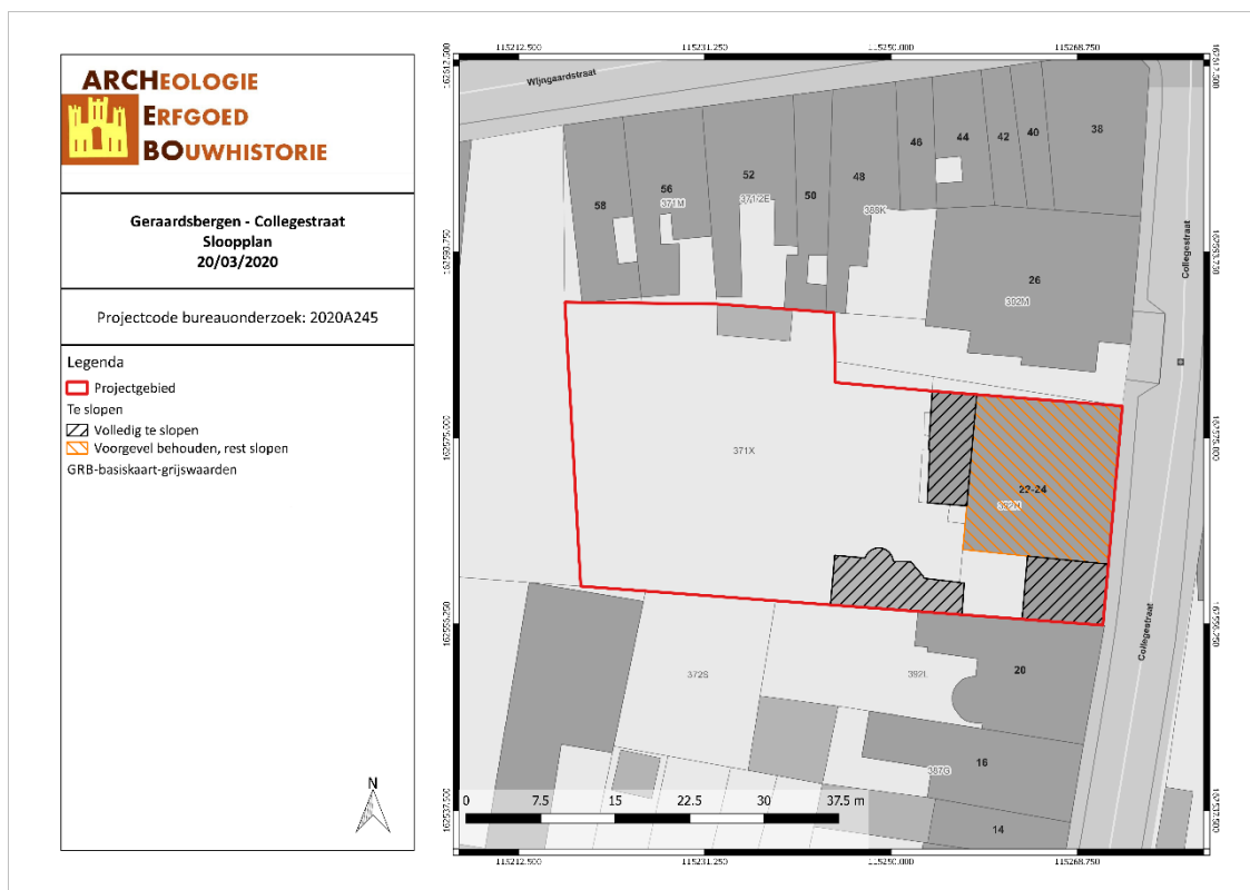
Figuur 20: Sloopplan (ARCHEBO bvba, 2020)
