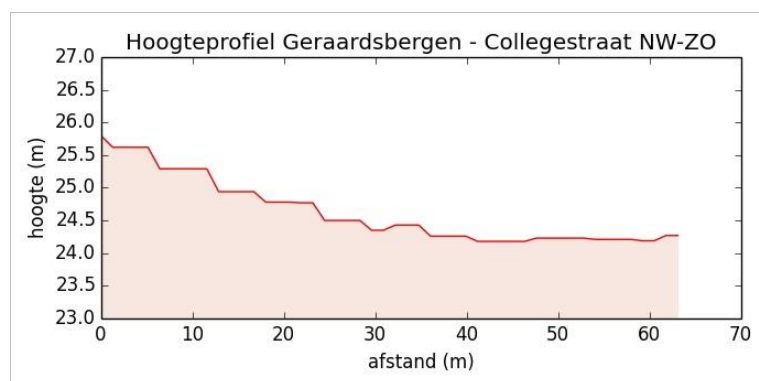
Figuur 26: Hoogteprofiel doorheen het plangebied in NW-ZO richting (Geopunt, 2020)
