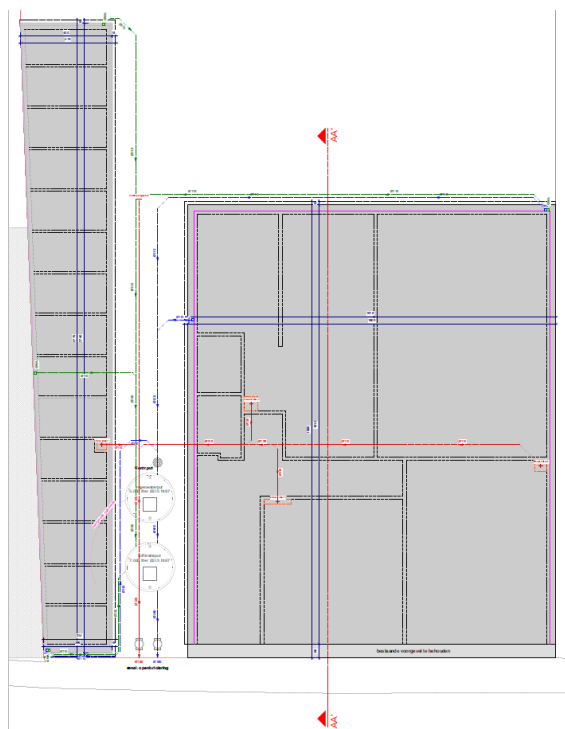
Figuur 15: Fundering (Drieskens & Dubois - architecten cvba, 2020)
