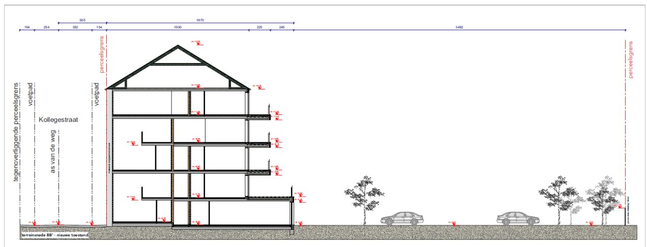
Figuur 17: Nieuw terreinprofiel (Drieskens & Dubois - architecten cvba, 2020)
