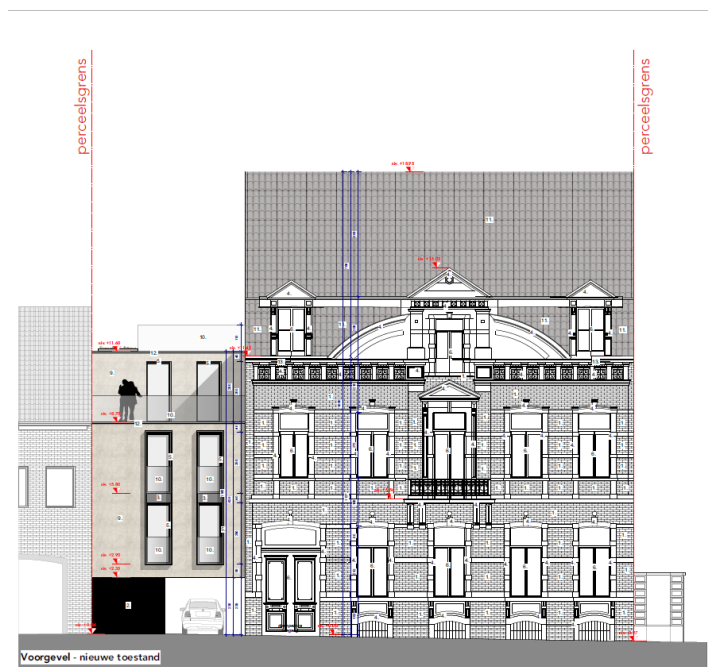
Figuur 18: Voorgevel nieuw (Drieskens & Dubois - architecten cvba, 2020)
