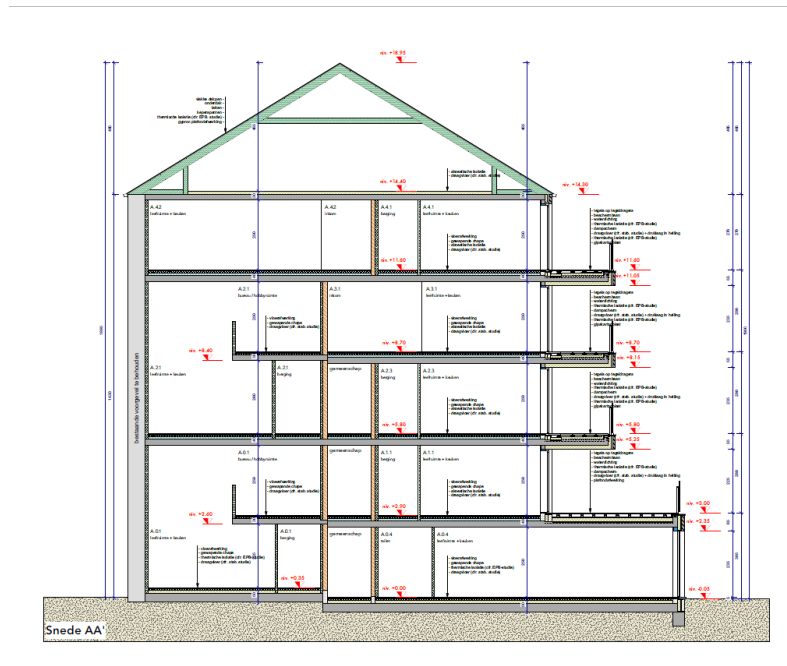
Figuur 16: Doorsnede (Drieskens & Dubois - architecten cvba, 2020)
