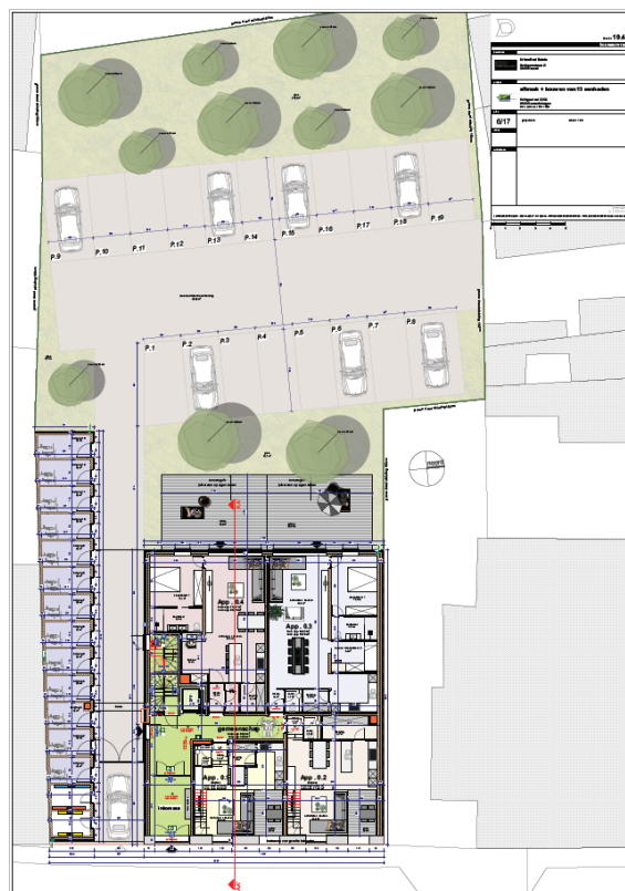
Figuur 14: Gelijkvloers (Drieskens & Dubois - architecten cvba, 2020)
