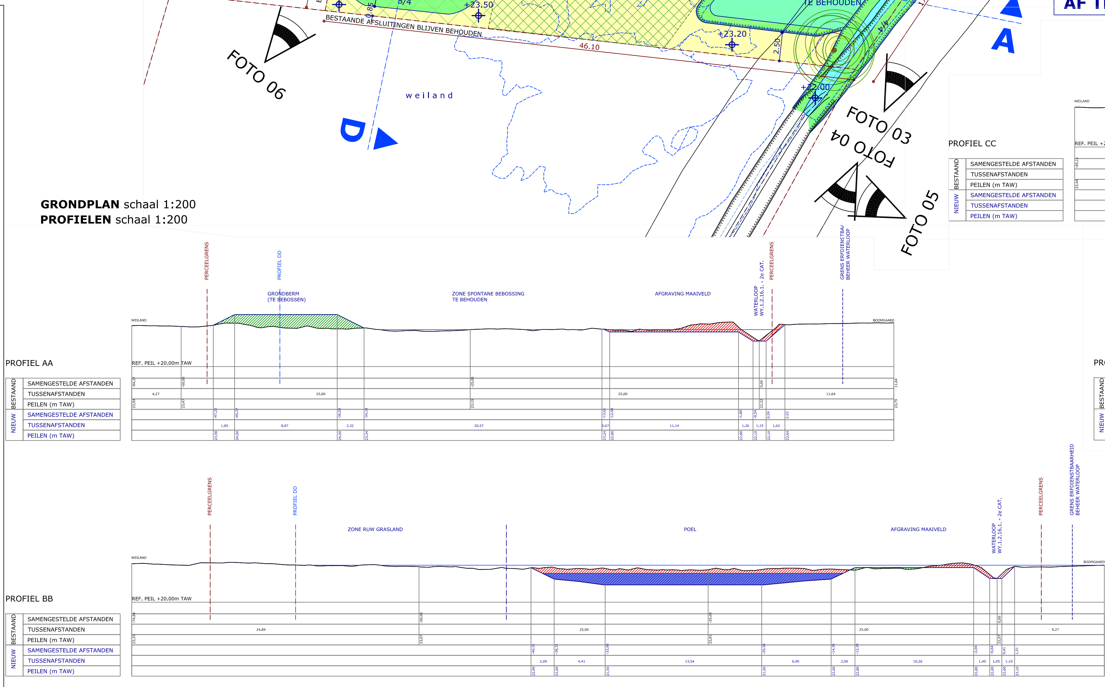
PROFIELEN schaal 1:200
