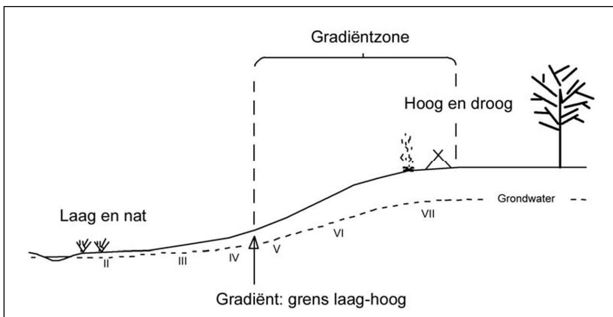
Afb. 26: Hypothetisch voorbeeld van een gradiëntzone (M. Verhoeven et al. 2010, Fig. 33, p.87)
